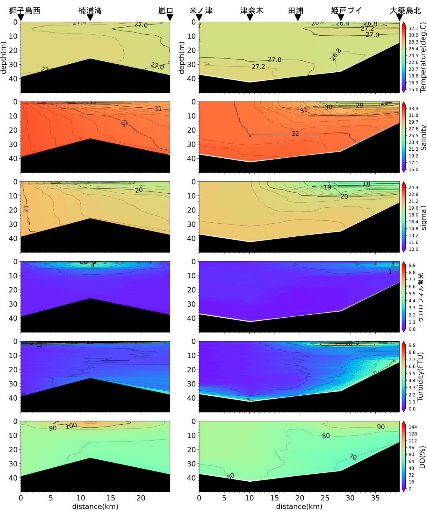
嵐口から獅子島西，大築島北から米ノ津の水温(°C)、塩分、密度( \sigma_t )、クロロフィル蛍光強度、濁度、溶存酸素飽和度(DO%)の鉛直面図(東町漁業協同組合の調査による)(2024年9月24日)
