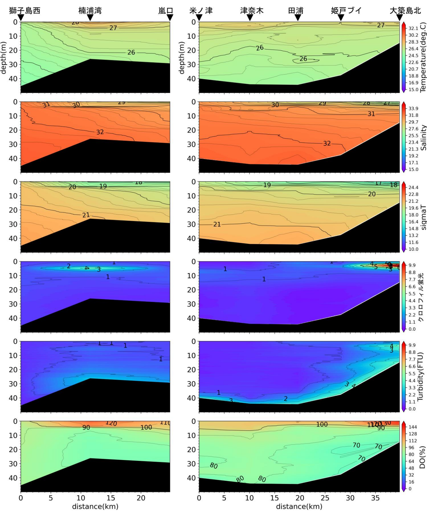
嵐口から獅子島西, 大築島北から米ノ津の水温(°C)、塩分、密度( \sigma_t )、クロロフィル蛍光強度、濁度、溶存酸素飽和度(DO%)の鉛直面図(東町漁業協同組合の調査による)(2024年9月3日)
