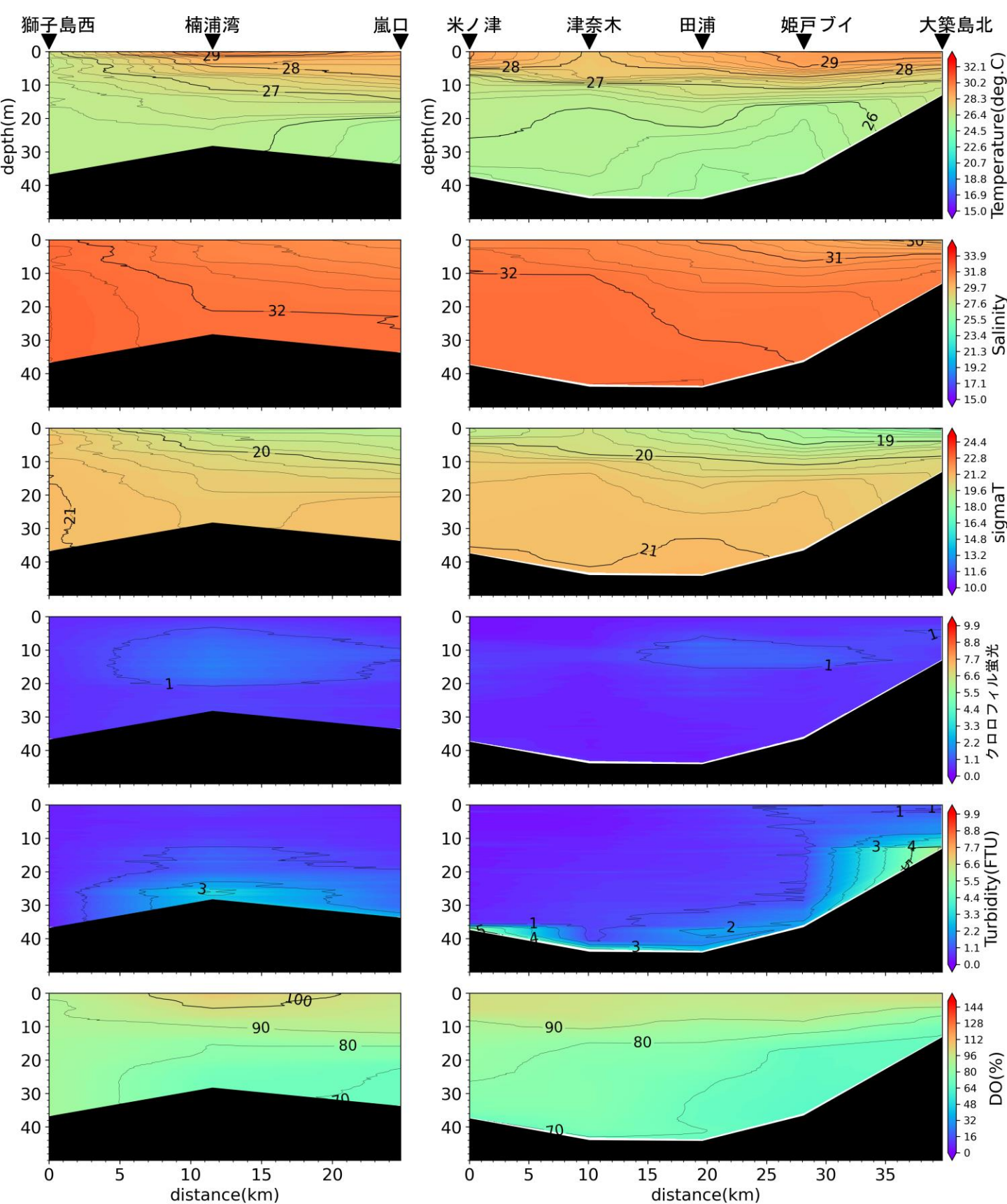
嵐口から獅子島西, 大築島北から米ノ津の水温(°C)、塩分、密度( \sigma_t )、クロロフィル蛍光強度、濁度、溶存酸素飽和度(DO%)の鉛直面図(東町漁業協同組合の調査による)(2024年8月26日)
