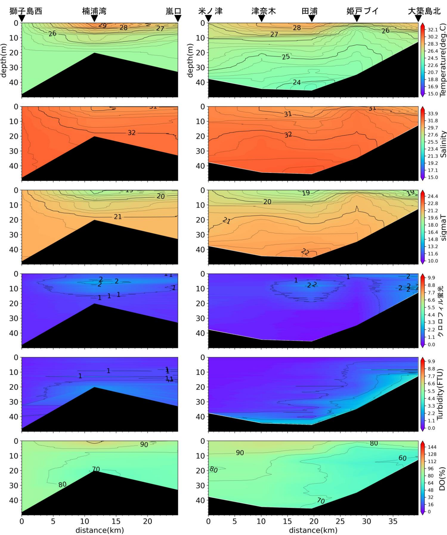
嵐口から獅子島西，大築島北から米ノ津の水温(°C)、塩分、密度( \sigma_t )、クロロフィル蛍光強度、濁度、溶存酸素飽和度(DO%)の鉛直面図(熊本県水産研究センターの調査による)(2024年8月20日)
