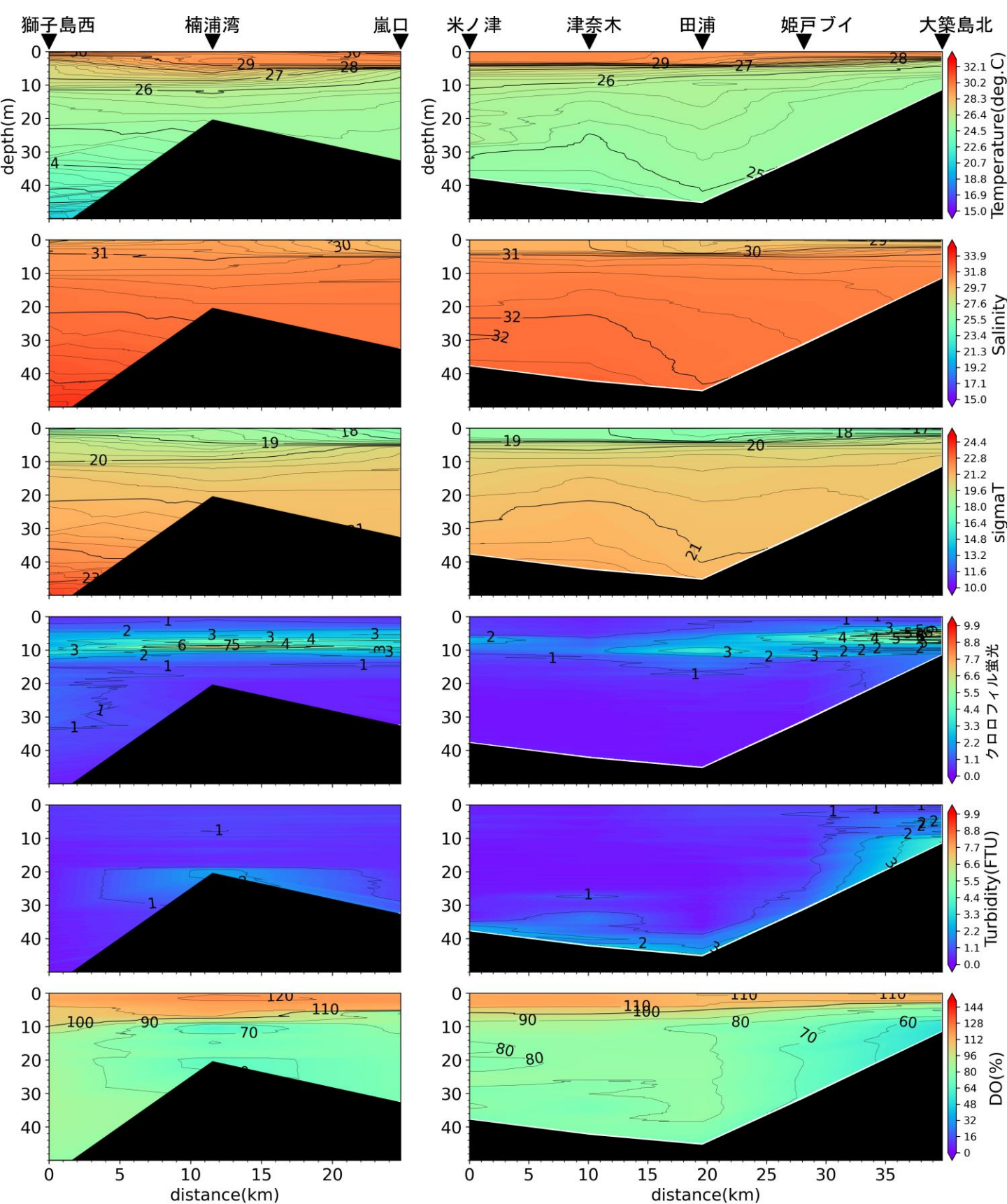
嵐口から獅子島西，大築島北から米ノ津の水温(°C)、塩分、密度( \sigma_t )、クロロフィル蛍光強度、濁度、溶存酸素飽和度(DO%)の鉛直面図(鹿児島県水産技術開発センターの調査による)(2024年8月14日)
