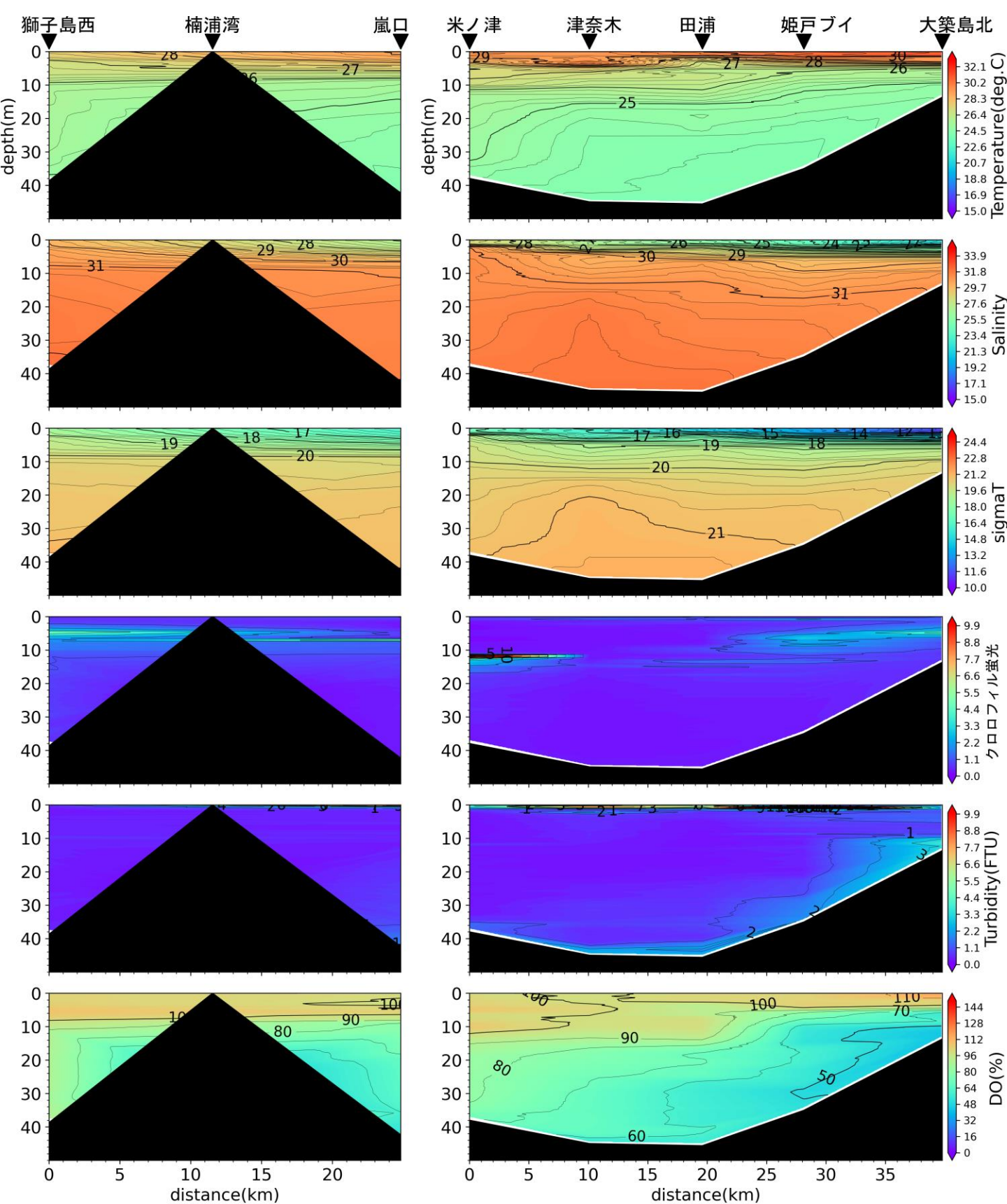
嵐口から獅子島西, 大築島北から米ノ津の水温(°C)、塩分、密度( \sigma_t )、クロロフィル蛍光強度、濁度、溶存酸素飽和度(DO%)の鉛直面図(東町漁業協同組合の調査による)(2024年7月30日)
