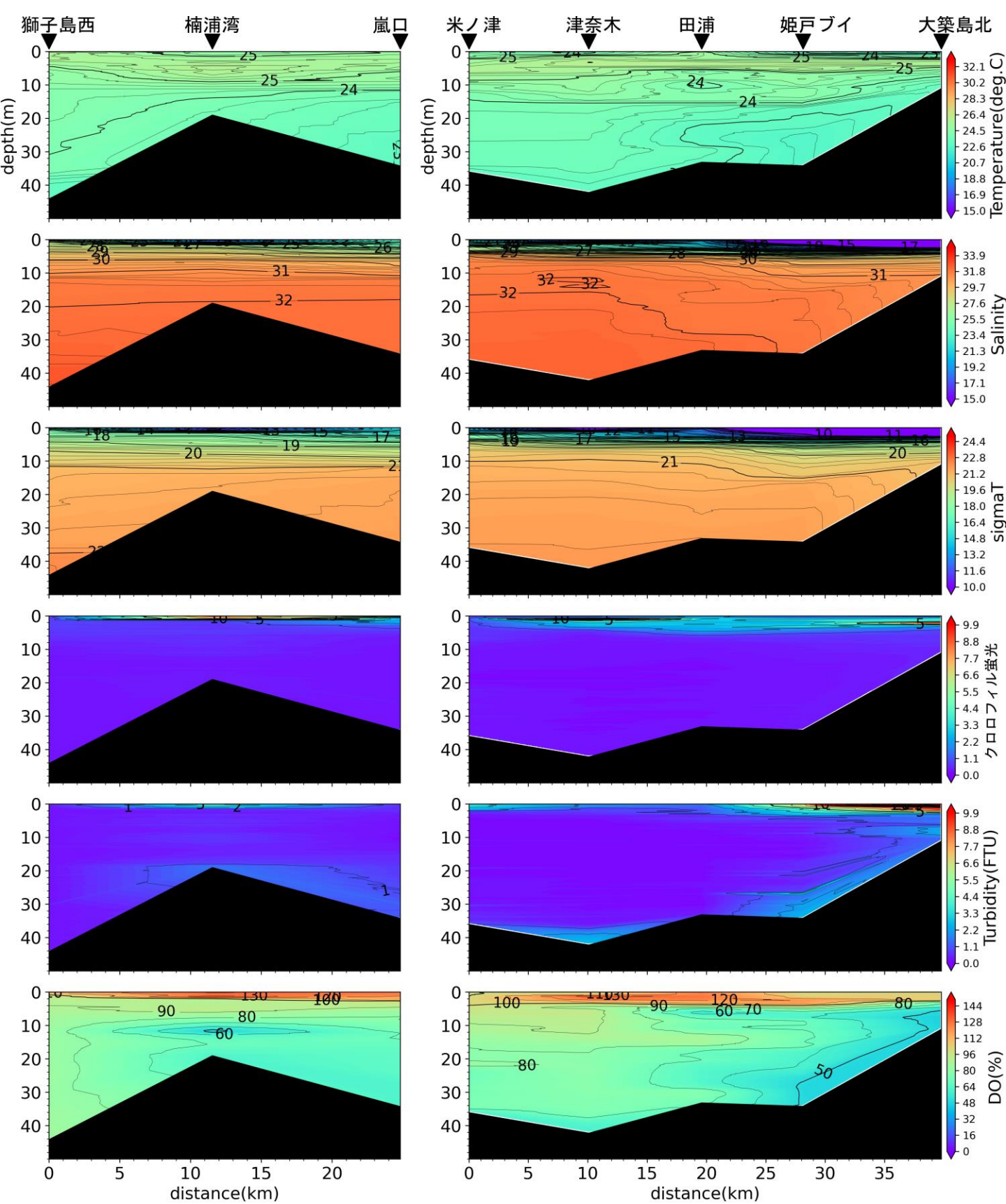
嵐口から獅子島西, 大築島北から米ノ津の水温(°C)、塩分、密度( \sigma_t )、クロロフィル蛍光強度、濁度、溶存酸素飽和度(DO%)の鉛直面図(熊本県水産研究センターの調査による)(2024年7月16日)
