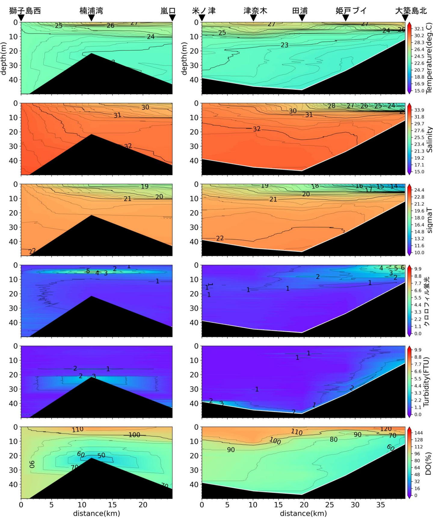
嵐口から獅子島西，大築島北から米ノ津の水温(°C)、塩分、密度( \sigma_t )、クロロフィル蛍光強度、濁度、溶存酸素飽和度(DO%)の鉛直面図(鹿児島県水産技術開発センターの調査による)(2024年7月9日)
