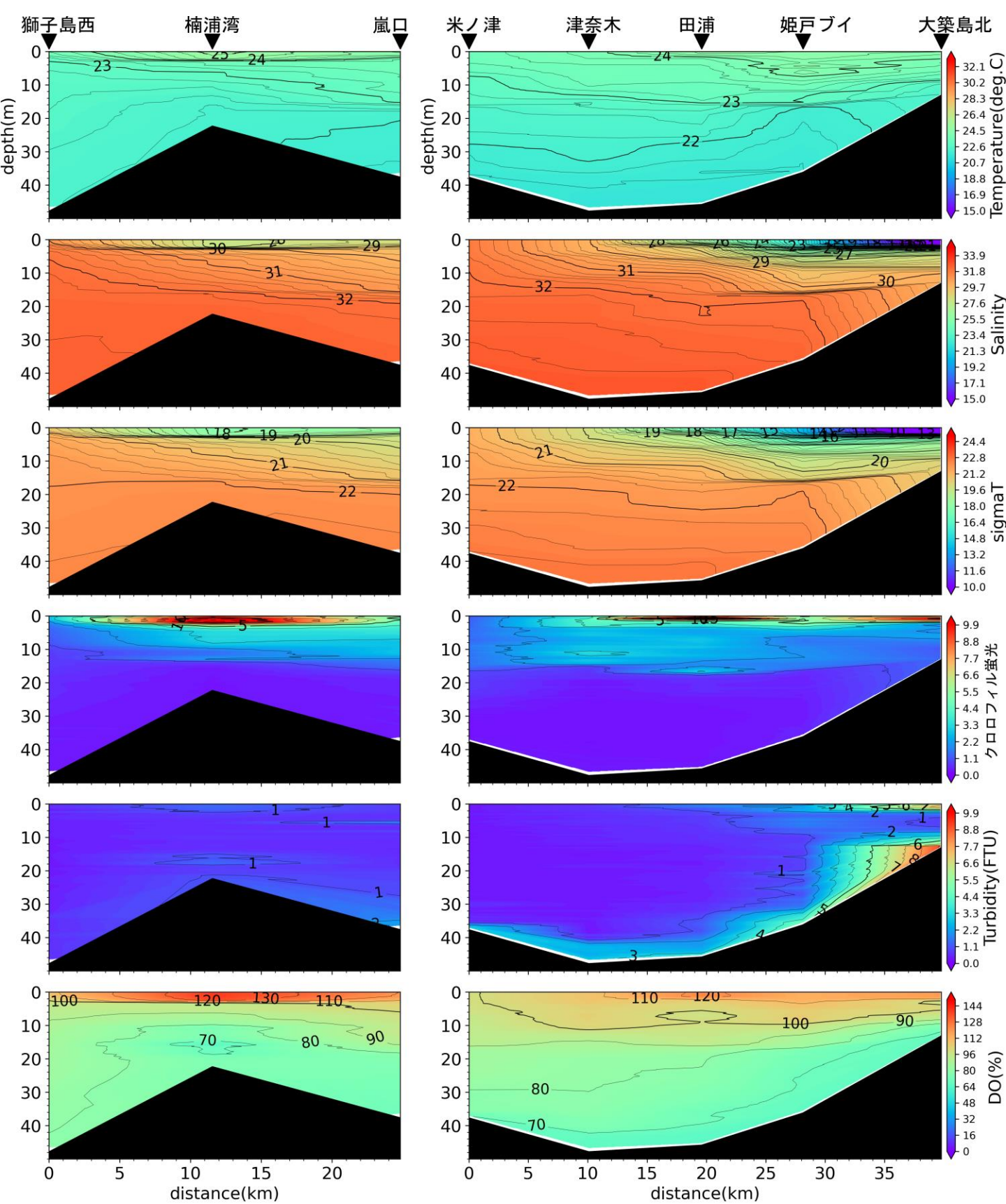
嵐口から獅子島西, 大築島北から米ノ津の水温(°C)、塩分、密度( \sigma_t )、クロロフィル蛍光強度、濁度、溶存酸素飽和度(DO%)の鉛直面図(東町漁業協同組合の調査による)(2024年7月2日)
