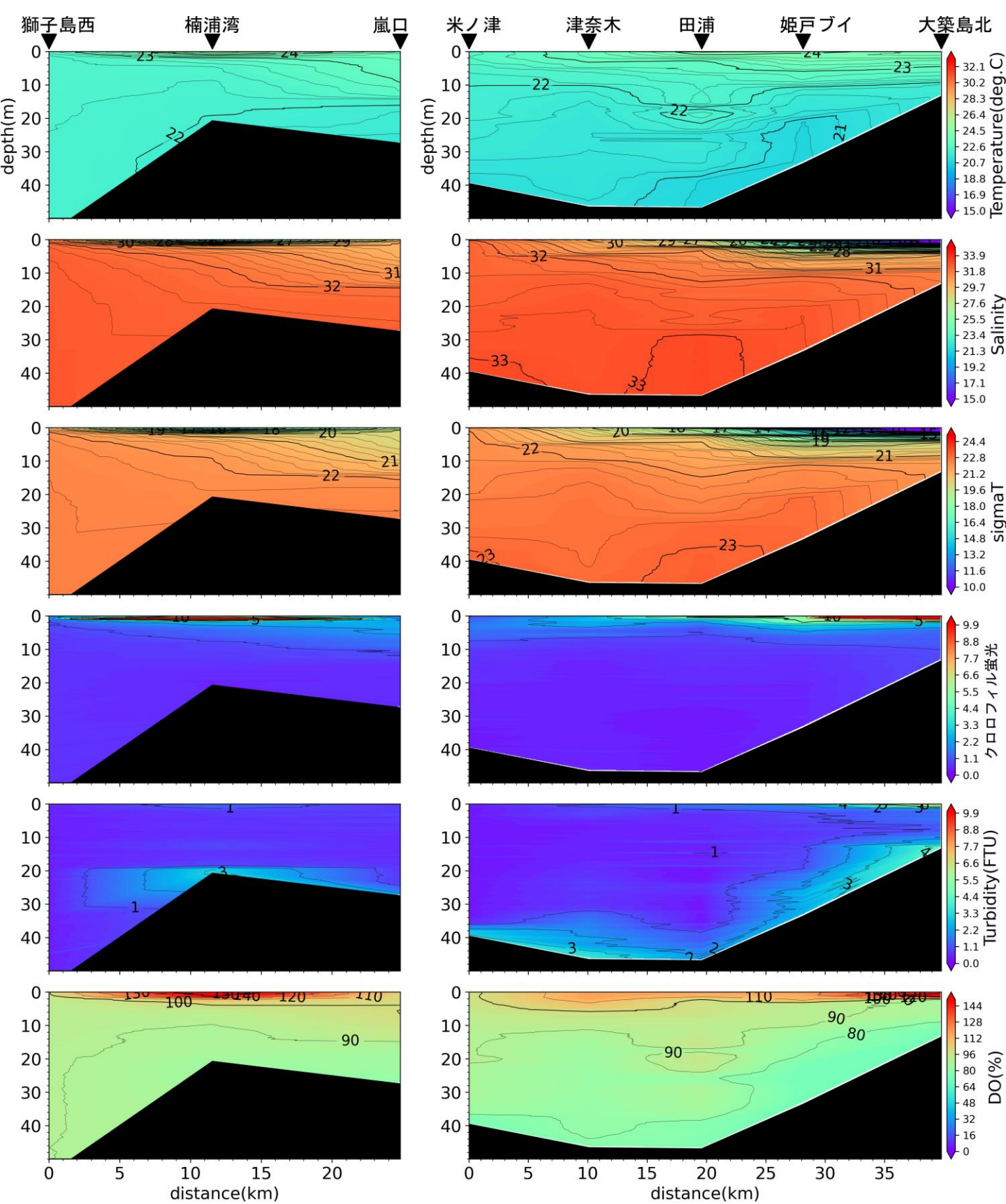
嵐口から獅子島西, 大築島北から米ノ津の水温(°C)、塩分、密度( \sigma_t )、クロロフィル蛍光強度、濁度、溶存酸素飽和度(DO%)の鉛直面図(鹿児島県水産技術開発センターの調査による)(2024年6月25日)
