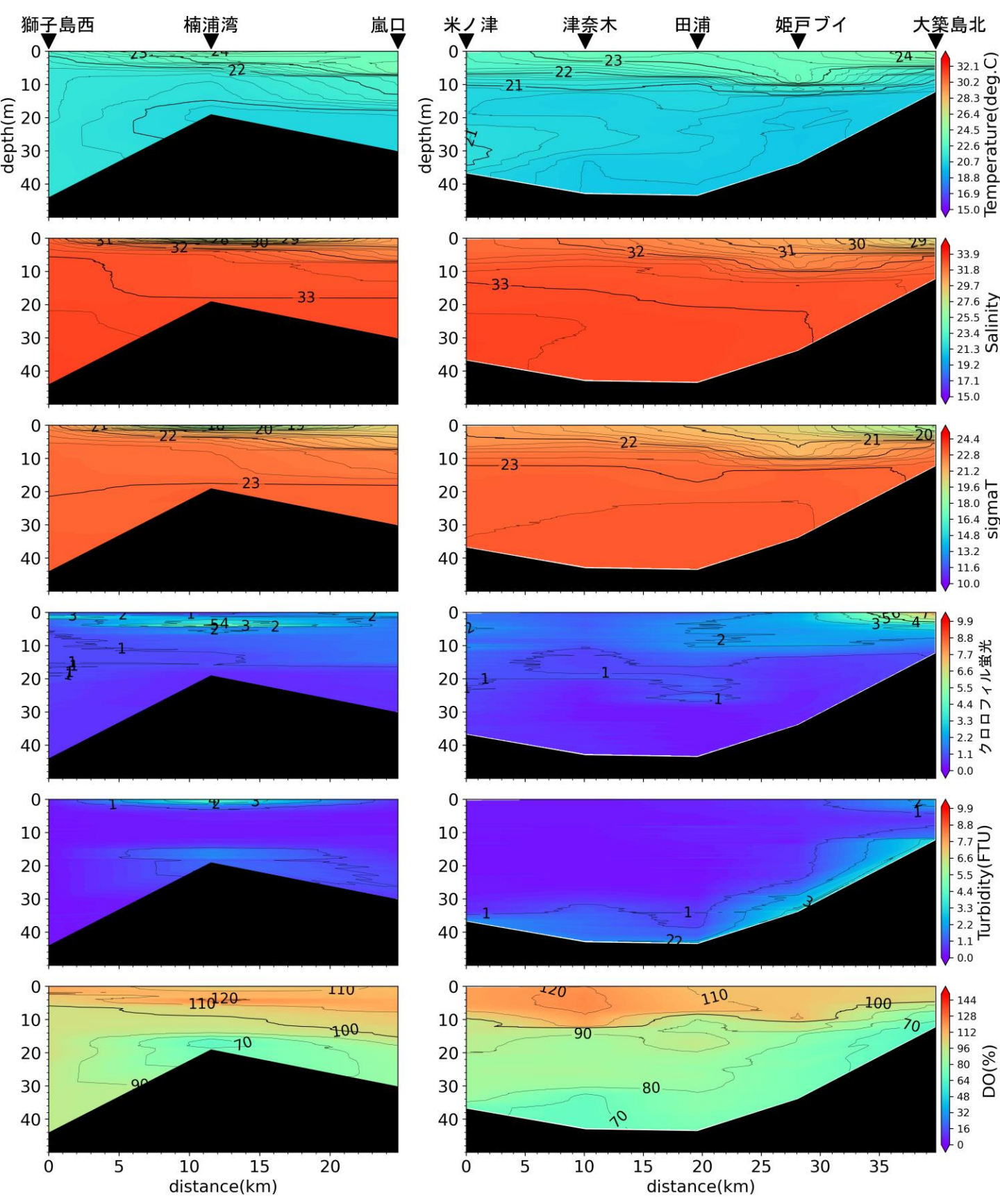
嵐口から獅子島西，大築島北から米ノ津の水温(°C)、塩分、密度( \sigma_t )、クロロフィル蛍光強度、濁度、溶存酸素飽和度(DO%)の鉛直面図(熊本県水産研究センターの調査による)(2024年6月18日)
