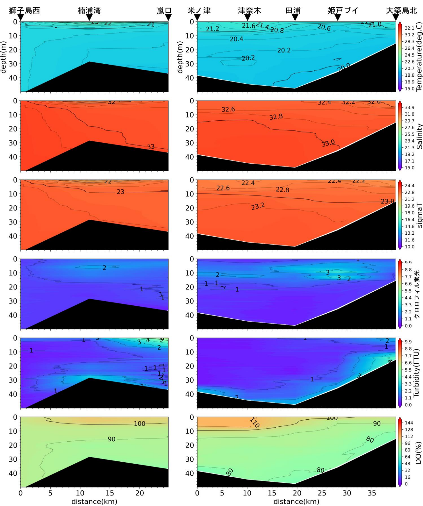
嵐口から獅子島西, 大築島北から米ノ津の水温(°C)、塩分、密度( \sigma_t )、クロロフィル蛍光強度、濁度、溶存酸素飽和度(DO%)の鉛直面図(東町漁業協同組合の調査による)(2024年6月11日)
