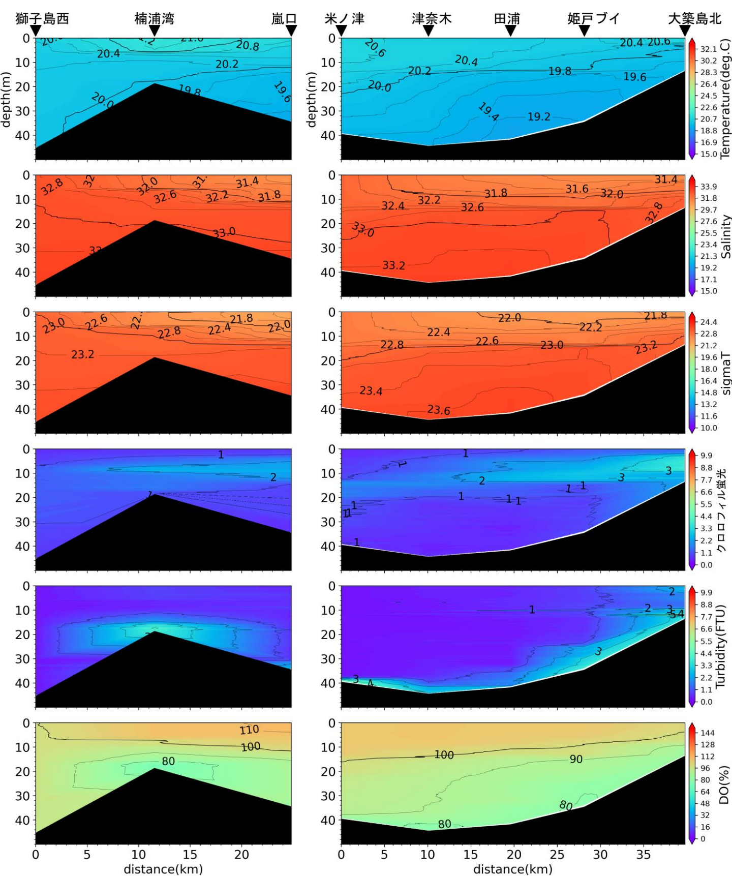
嵐口から獅子島西，大築島北から米ノ津の水温(°C)、塩分、密度( \sigma_t )、クロロフィル蛍光強度、濁度、溶存酸素飽和度(DO%)の鉛直面図(鹿児島県水産技術開発センターの調査による)(2024年6月4日)
