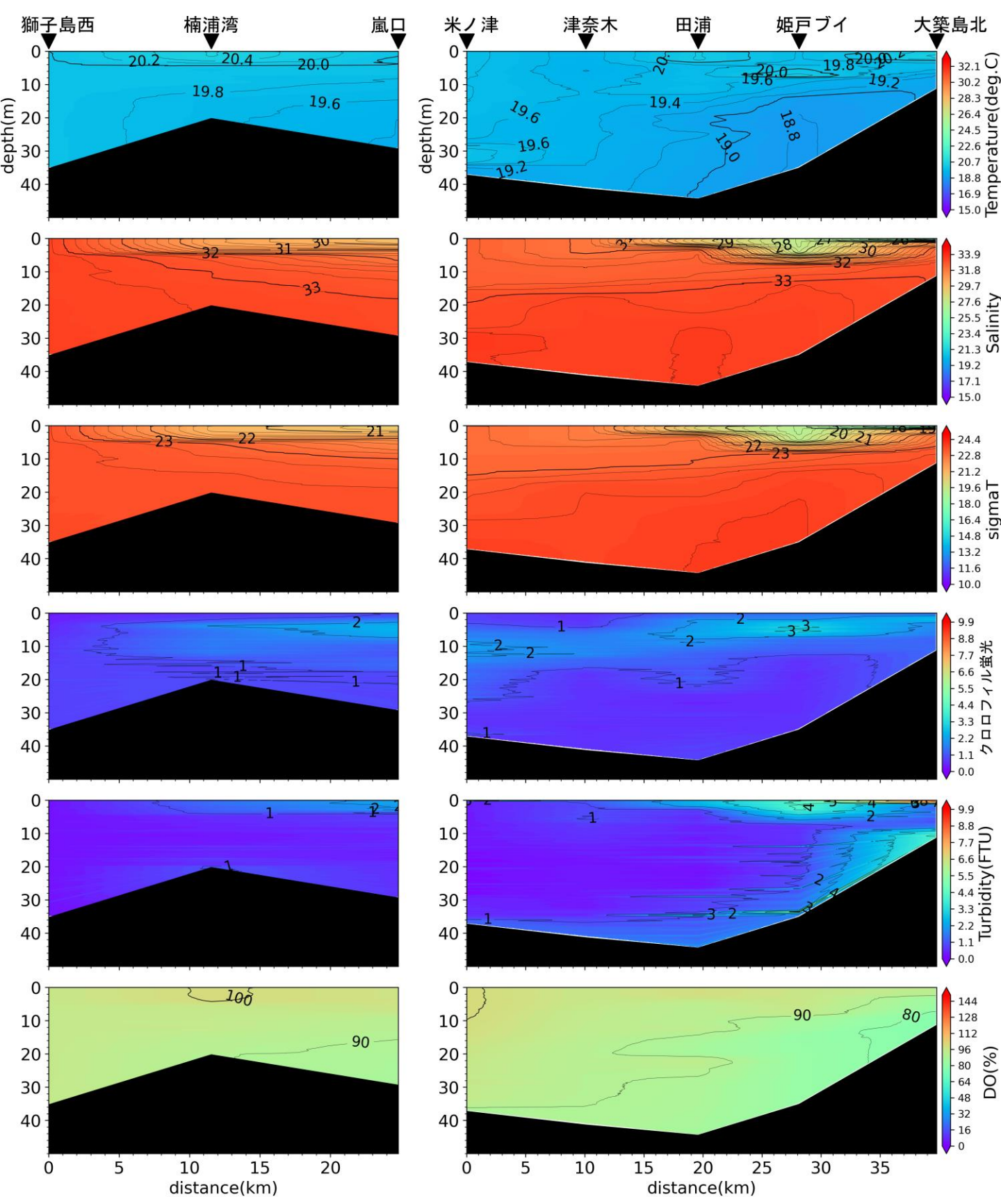
嵐口から獅子島西，大築島北から米ノ津の水温(°C)、塩分、密度( \sigma_t )、クロロフィル蛍光強度、濁度、溶存酸素飽和度(DO%)の鉛直面図(熊本県水産研究センターの調査による)(2024年5月29日)
