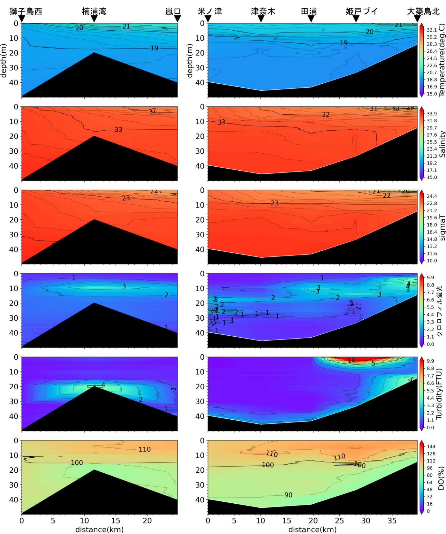
嵐口から獅子島西, 大築島北から米ノ津の水温(°C)、塩分、密度( \sigma_t )、クロロフィル蛍光強度、濁度、溶存酸素飽和度(DO%)の鉛直面図(鹿児島県水産技術開発センターの調査による)(2024年5月21日)
