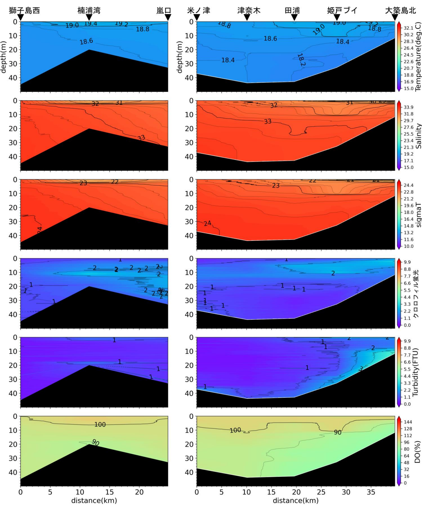
嵐口から獅子島西，大築島北から米ノ津の水温(°C)、塩分、密度( \sigma_t )、クロロフィル蛍光強度、濁度、溶存酸素飽和度(DO%)の鉛直面図(熊本県水産研究センターの調査による)(2024年5月14日)
