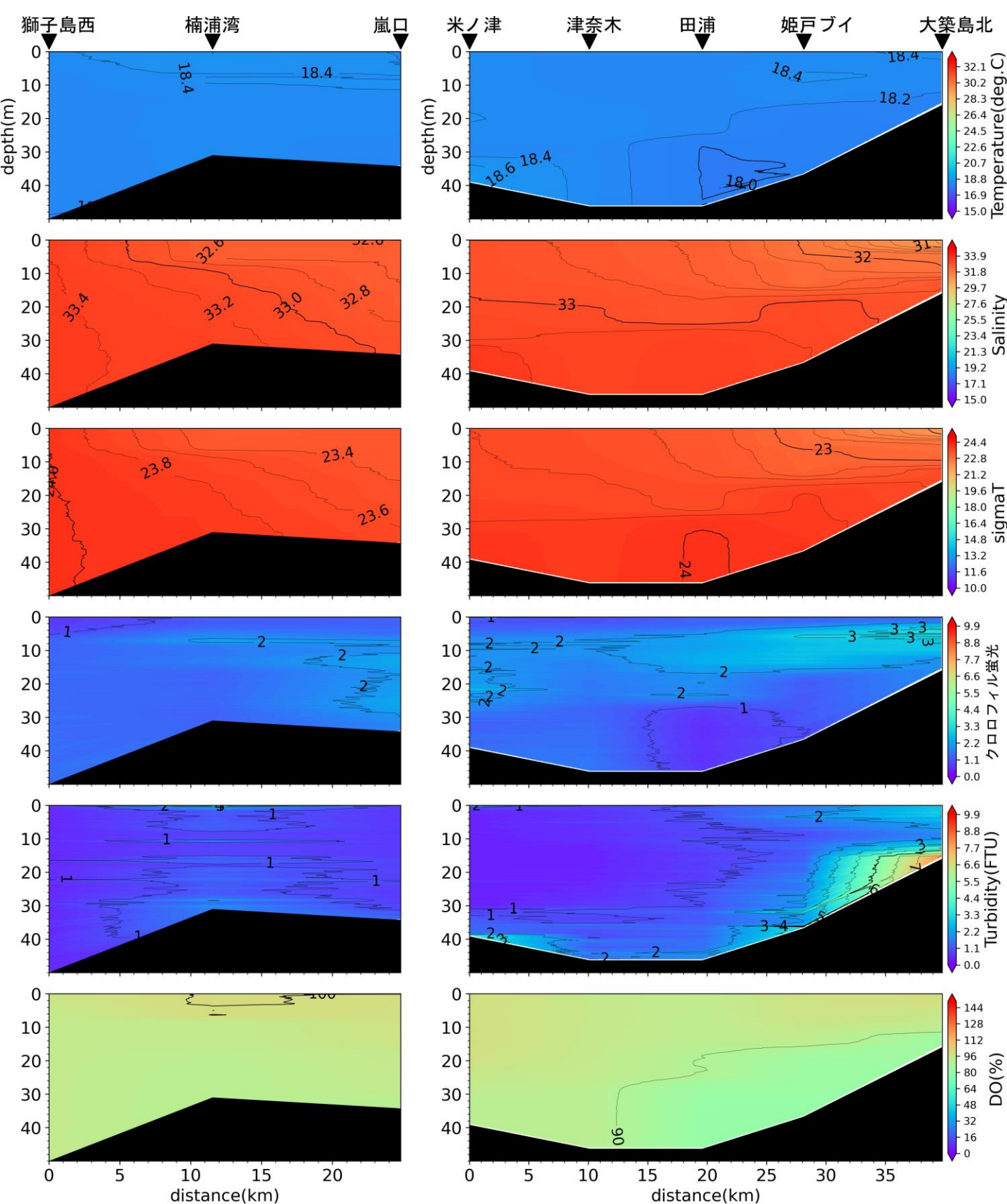
嵐口から獅子島西, 大築島北から米ノ津の水温(°C)、塩分、密度( \sigma_t )、クロロフィル蛍光強度、濁度、溶存酸素飽和度(DO%)の鉛直面図(東町漁業協同組合の調査による)(2024年5月9日)
