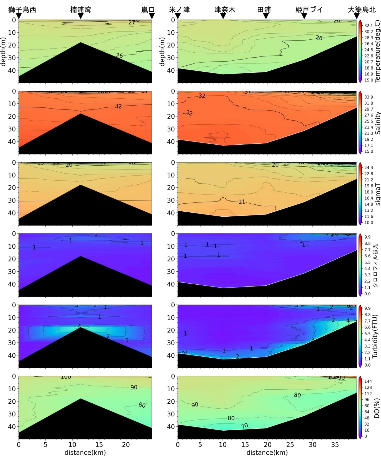
嵐口から獅子島西, 大築島北から米ノ津の水温(°C)、塩分、密度( \sigma_t )、クロロフィル蛍光強度、濁度、溶存酸素飽和度(DO%)の鉛直面図(鹿児島県水産技術開発センターの調査による)(2023年8月11日)
