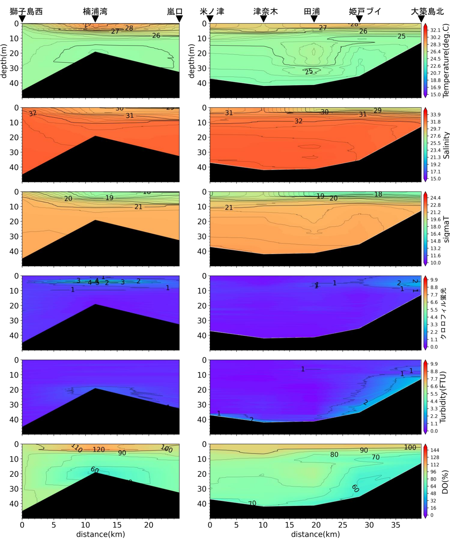
嵐口から獅子島西，大築島北から米ノ津の水温(°C)、塩分、密度( \sigma_t )、クロロフィル蛍光強度、濁度、溶存酸素飽和度(DO%)の鉛直面図(熊本県水産研究センターの調査による)(2023年8月1日)
