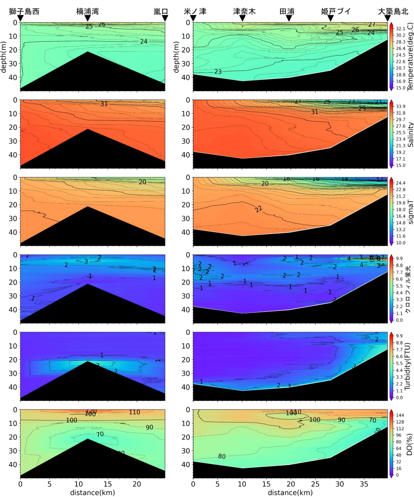
嵐口から獅子島西，大築島北から米ノ津の水温(°C)、塩分、密度( \sigma_t )、クロロフィル蛍光強度、濁度、溶存酸素飽和度(DO%)の鉛直面図(鹿児島県水産技術開発センターの調査による)(2023年7月11日)
