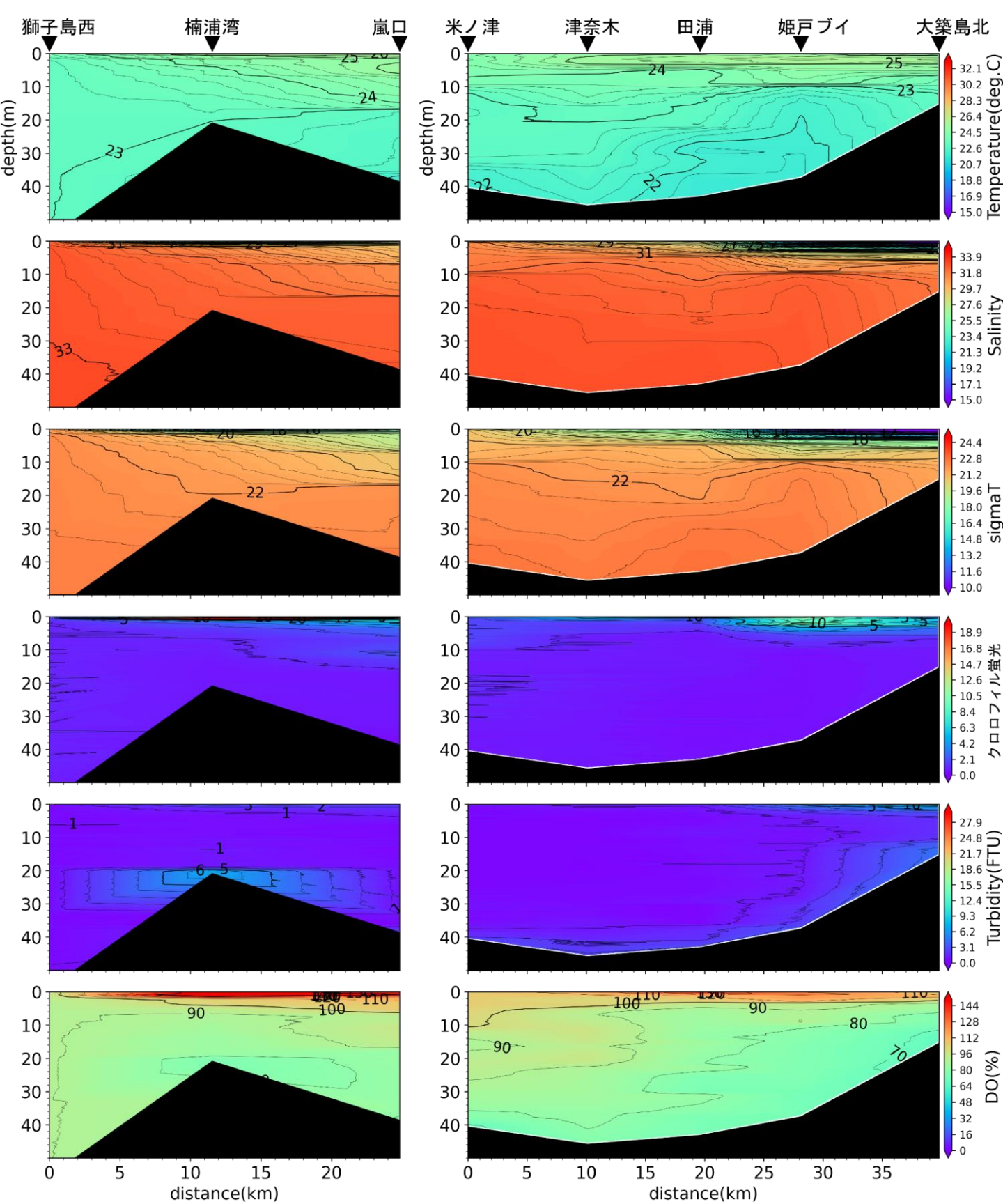
嵐口から獅子島西，大築島北から米ノ津の水温(°C)、塩分、密度( \sigma_t )、クロロフィル蛍光強度、濁度、溶存酸素飽和度(DO%)の鉛直面図(鹿児島県水産技術開発センターの調査による)(2023年7月4日)
