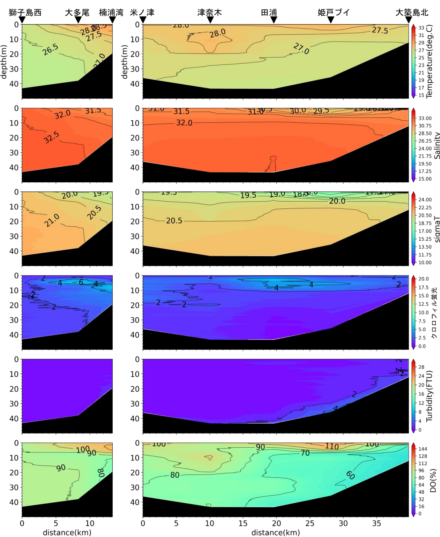
楠浦湾から獅子島西, 大築島北から米ノ津の水温(°C)、塩分、密度( \sigma_t )、クロロフィル蛍光強度、濁度、溶存酸素飽和度(DO%)の鉛直面図(熊本県水産研究センターの調査による)(2022年8月30日)
