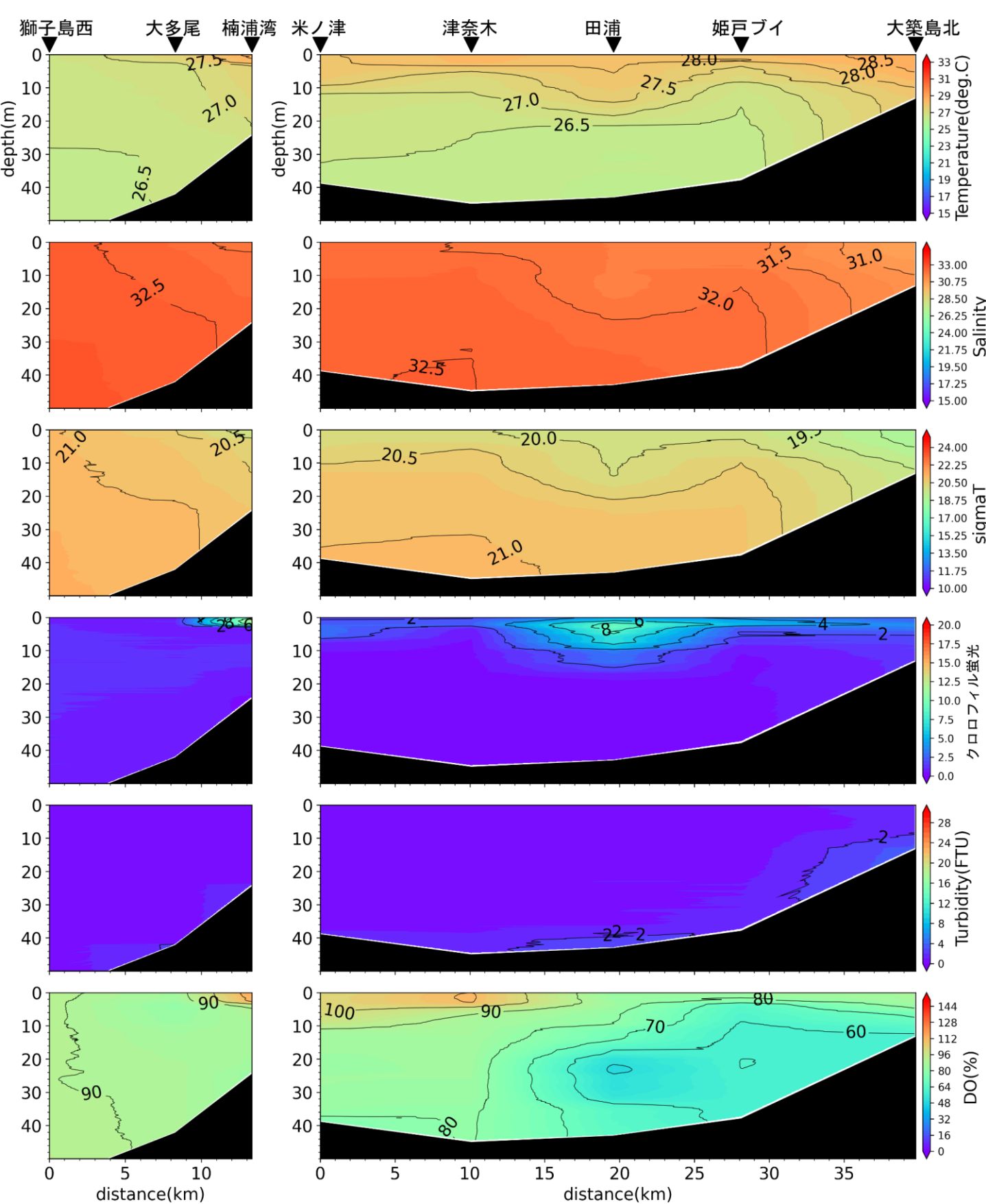
楠浦湾から獅子島西, 大築島北から米ノ津の水温(°C)、塩分、密度( \sigma_t )、クロロフィル蛍光強度、濁度、溶存酸素飽和度(DO%)の鉛直面図(鹿児島県水産技術開発センターの調査による)(2022年8月16日)
