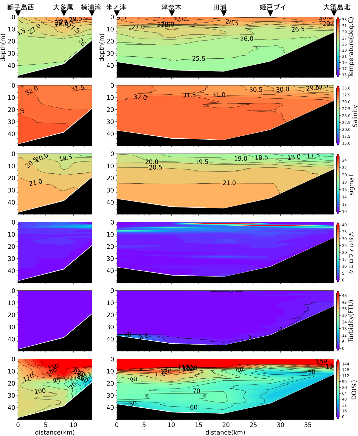
楠浦湾から獅子島西, 大築島北から米ノ津の水温(°C)、塩分、密度( \sigma_t )、クロロフィル蛍光強度、濁度、溶存酸素飽和度(DO%)の鉛直面図(熊本県水産研究センターの調査による)(2022年8月9日)
