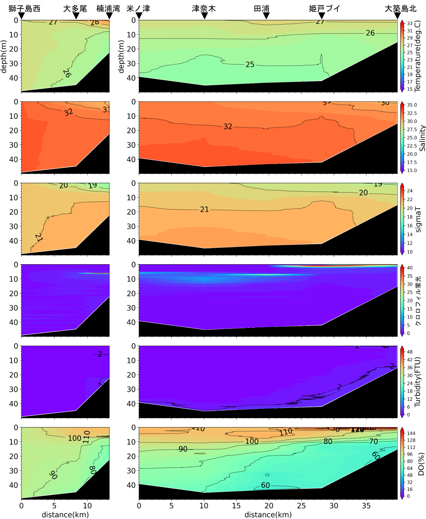
楠浦湾から獅子島西, 大築島北から米ノ津の水温(°C)、塩分、密度( \sigma_t )、クロロフィル蛍光強度、濁度、溶存酸素飽和度(DO%)の鉛直面図(鹿児島県水産技術開発センターの調査による)(2022年8月2日)
