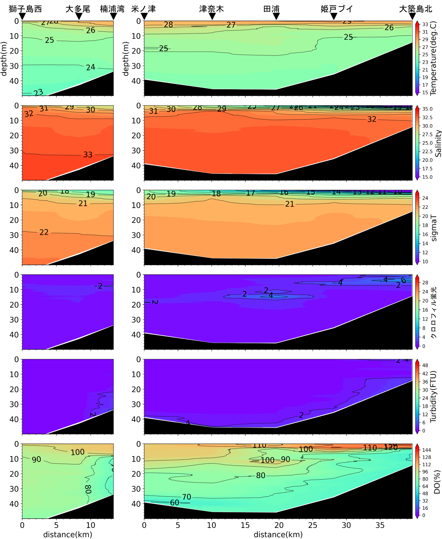
楠浦湾から獅子島西, 大築島北から米ノ津の水温(°C)、塩分、密度( \sigma_t )、クロロフィル蛍光強度、濁度、溶存酸素飽和度(DO%)の鉛直面図(東町漁業協同組合の調査による)(2022年7月26日)
