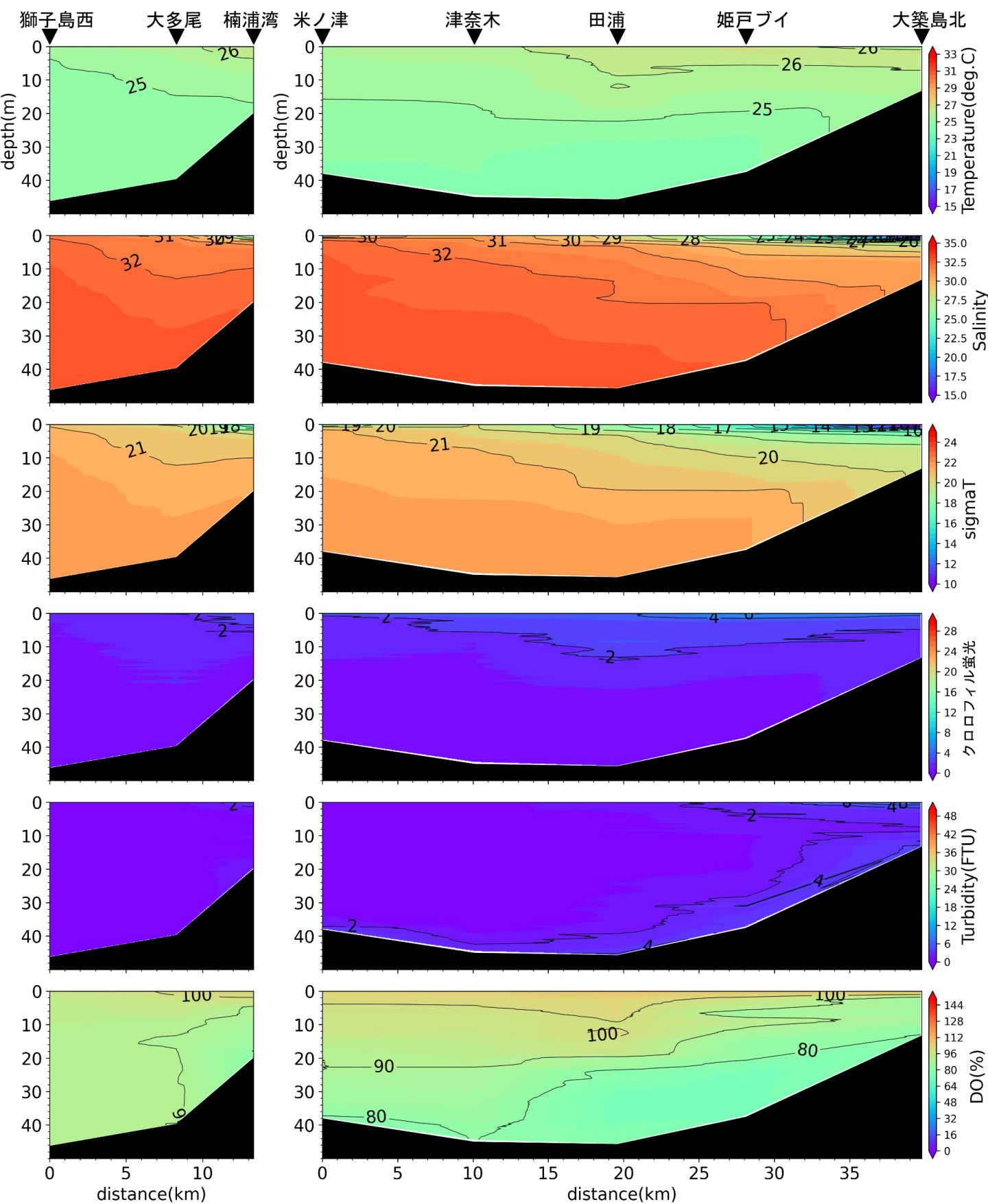
楠浦湾から獅子島西, 大築島北から米ノ津の水温(°C)、塩分、密度( \sigma_t )、クロロフィル蛍光強度、濁度、溶存酸素飽和度(DO%)の鉛直面図(熊本県水産研究センターの調査による)(2022年7月20日)
