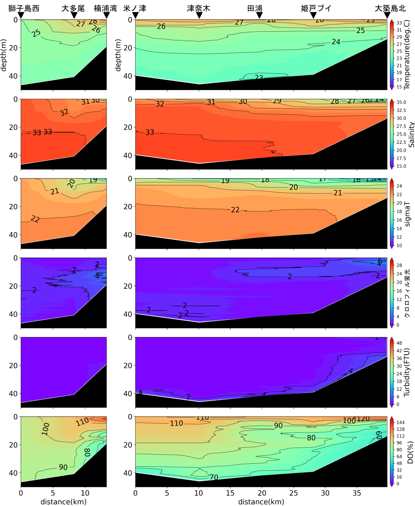
楠浦湾から獅子島西, 大築島北から米ノ津の水温(°C)、塩分、密度( \sigma_t )、クロロフィル蛍光強度、濁度、溶存酸素飽和度(DO%)の鉛直面図(鹿児島県水産技術開発センターの調査による)(2022年7月12日)
