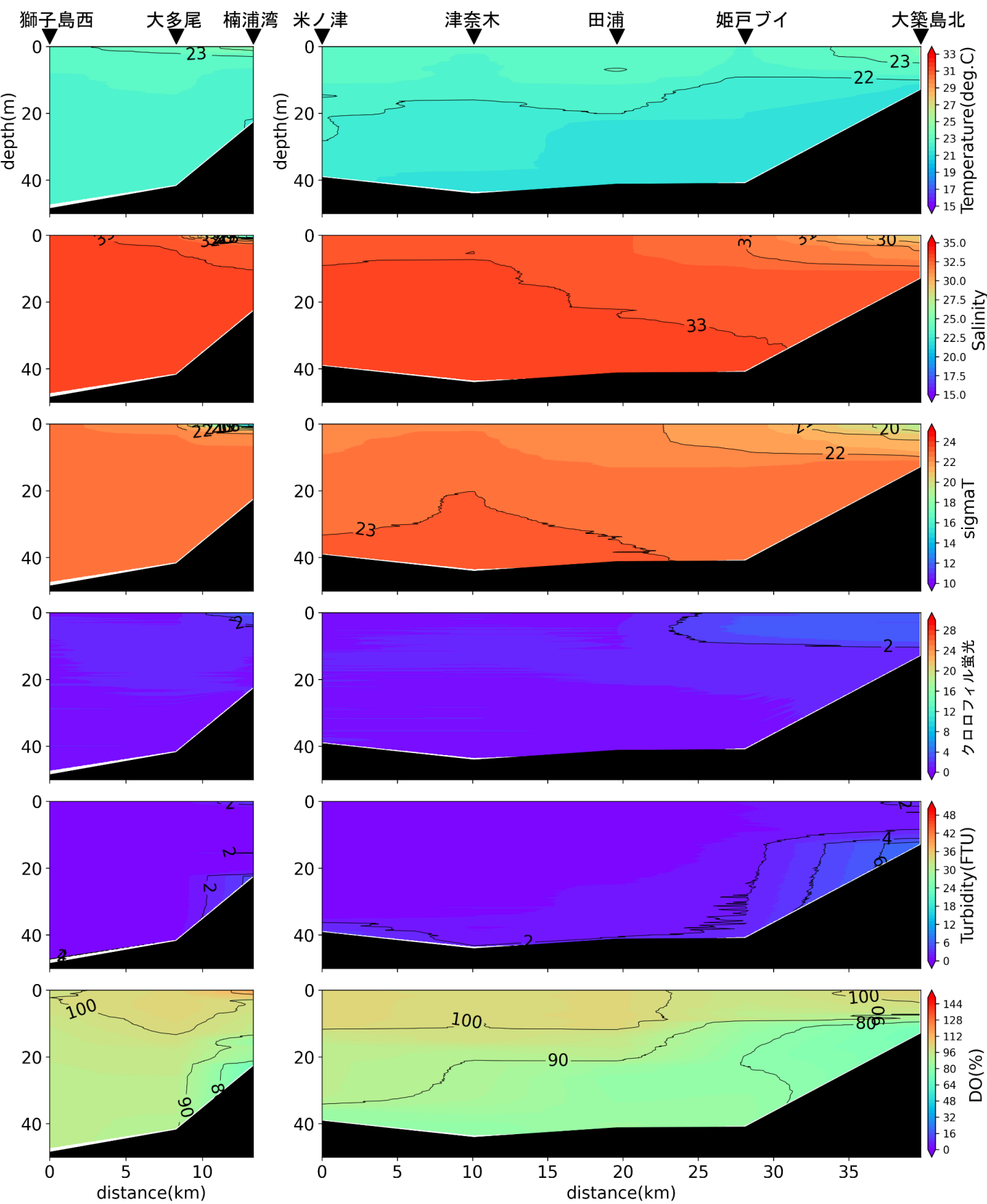
楠浦湾から獅子島西, 大築島北から米ノ津の水温(°C)、塩分、密度( \sigma_t )、クロロフィル蛍光強度、濁度、溶存酸素飽和度(DO%)の鉛直面図(鹿児島県水産技術開発センターの調査による)(2022年6月22日)
