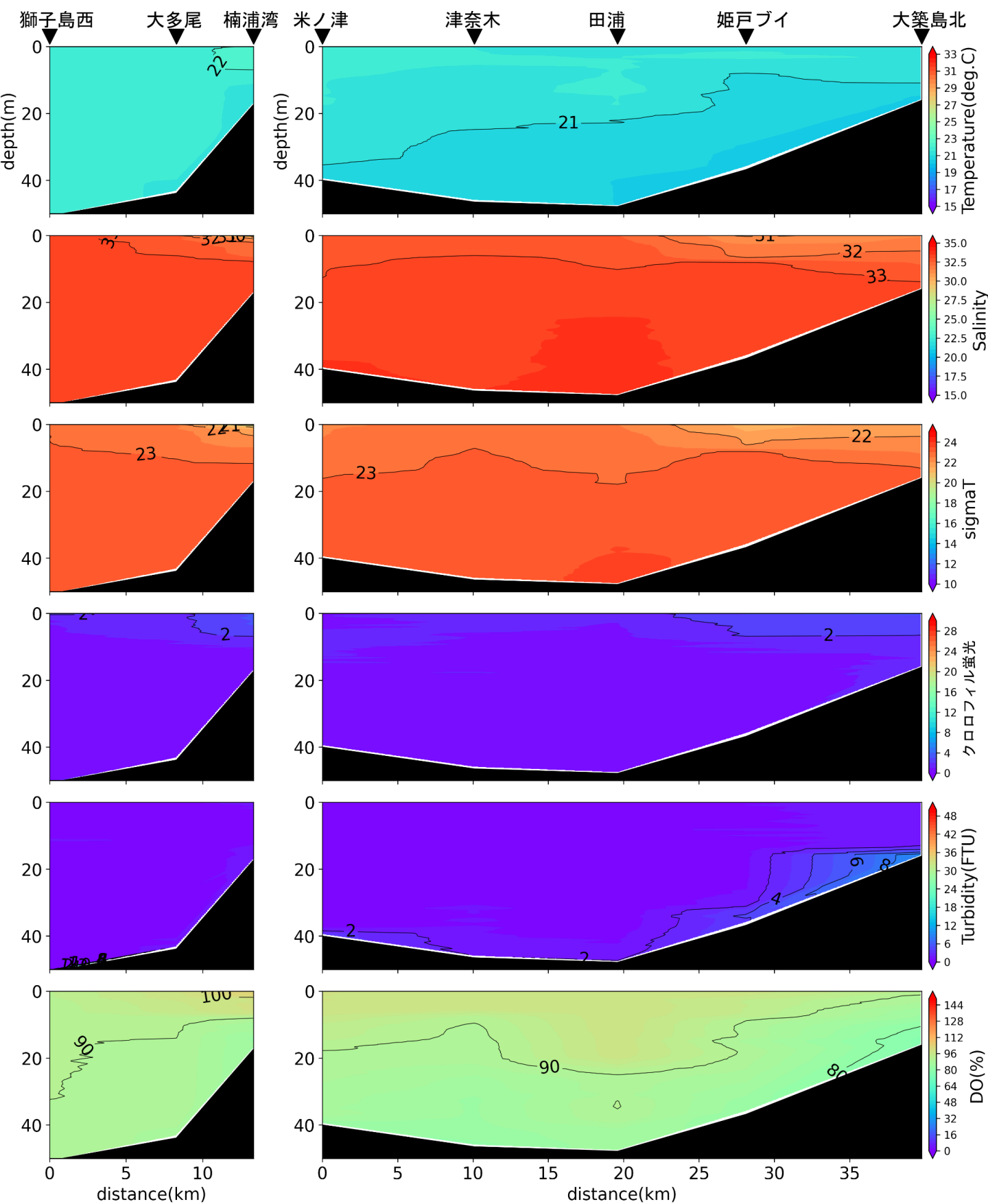
楠浦湾から獅子島西, 大築島北から米ノ津の水温(°C)、塩分、密度( \sigma_t )、クロロフィル蛍光強度、濁度、溶存酸素飽和度(DO%)の鉛直面図(東町漁業協同組合の調査による)(2022年6月14日)
