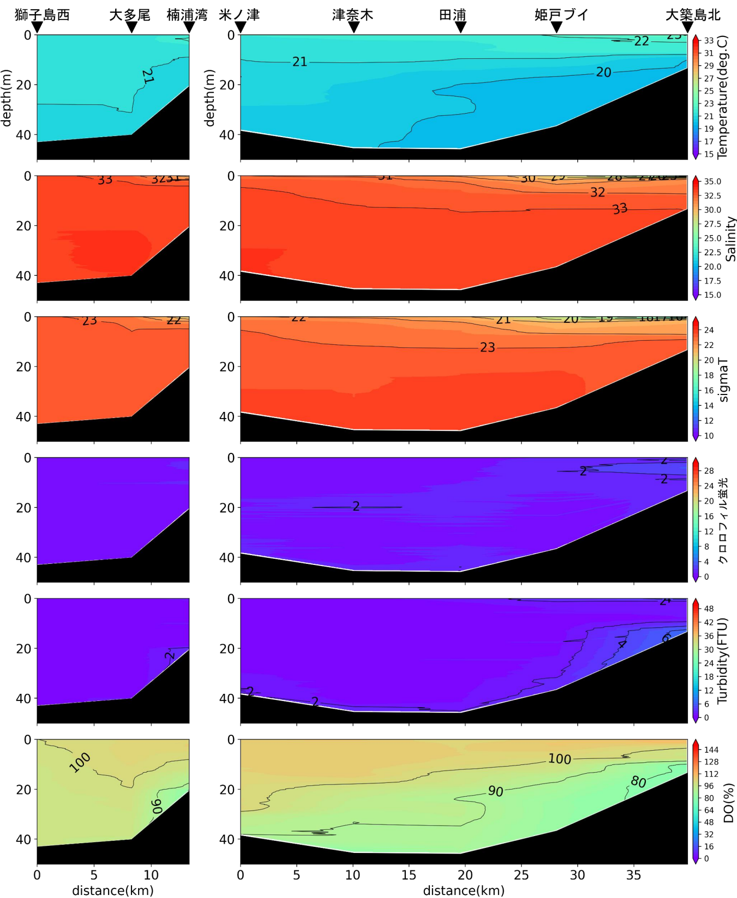
楠浦湾から獅子島西, 大築島北から米ノ津の水温(°C)、塩分、密度( \sigma_t )、クロロフィル蛍光強度、濁度、溶存酸素飽和度(DO%)の鉛直面図(熊本県水産研究センターの調査による)(2022年6月7日)
