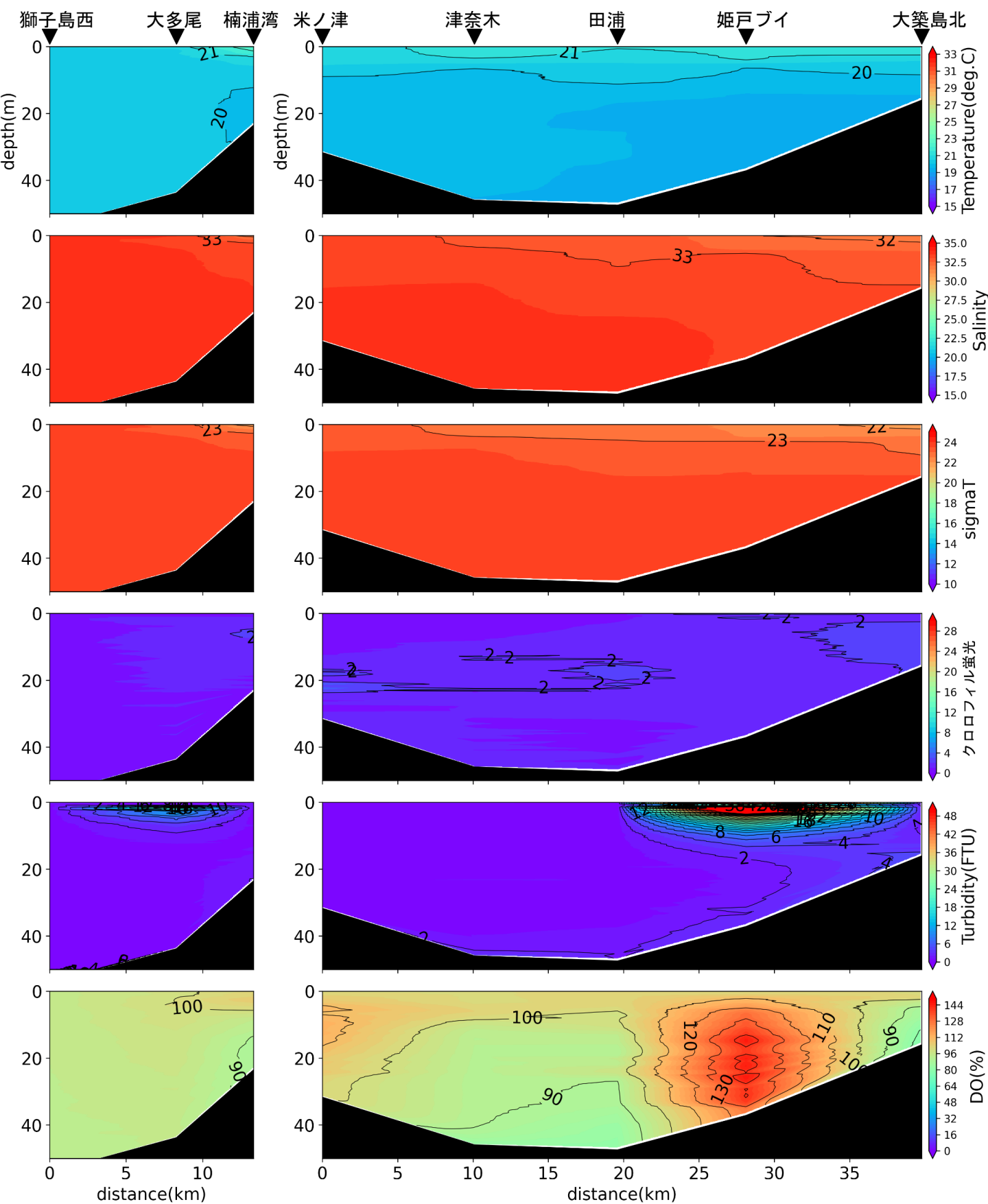
楠浦湾から獅子島西, 大築島北から米ノ津の水温( ^{\circ}\text{C} )、塩分、密度( \sigma_t )、クロロフィル蛍光強度、濁度、溶存酸素飽和度(DO%)の鉛直面図(東町漁業協同組合の調査による)(2022年5月31日)
