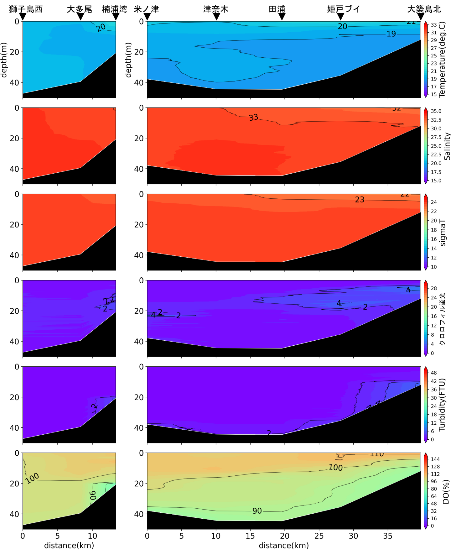
楠浦湾から獅子島西, 大築島北から米ノ津の水温(°C)、塩分、密度( \sigma_t )、クロロフィル蛍光強度、濁度、溶存酸素飽和度(DO%)の鉛直面図(熊本県水産研究センターの調査による)(2022年5月24日)
