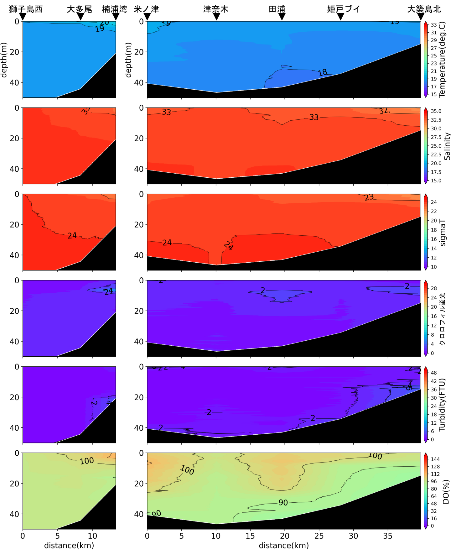
楠浦湾から獅子島西, 大築島北から米ノ津の水温(°C)、塩分、密度( \sigma_t )、クロロフィル蛍光強度、濁度、溶存酸素飽和度(DO%)の鉛直面図(鹿児島県水産技術開発センターの調査による)(2022年5月17日)
