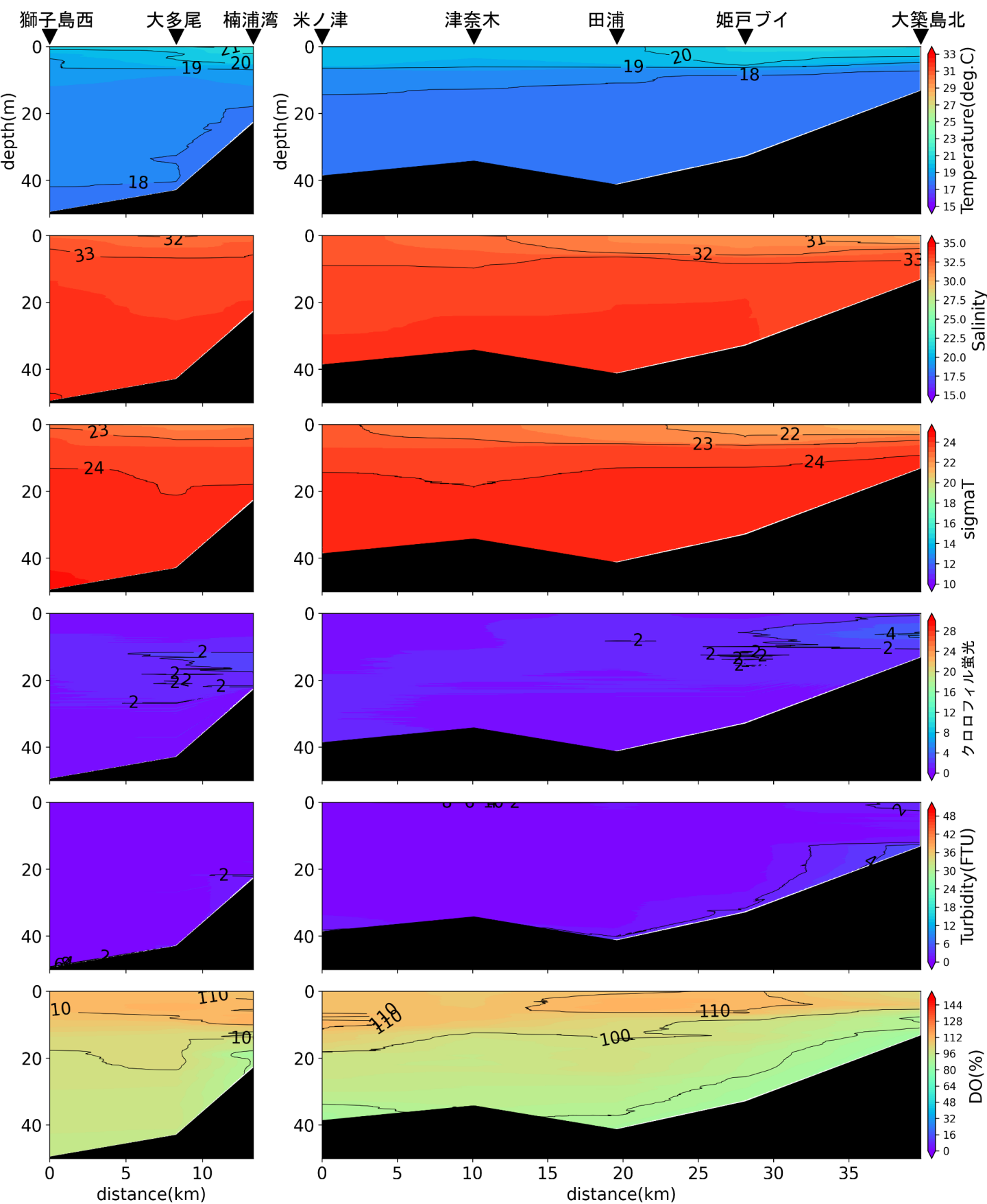
楠浦湾から獅子島西, 大築島北から米ノ津の水温(°C)、塩分、密度( \sigma_t )、クロロフィル蛍光強度、濁度、溶存酸素飽和度(DO%)の鉛直面図(鹿児島県水産技術開発センターの調査による)(2022年5月10日)
