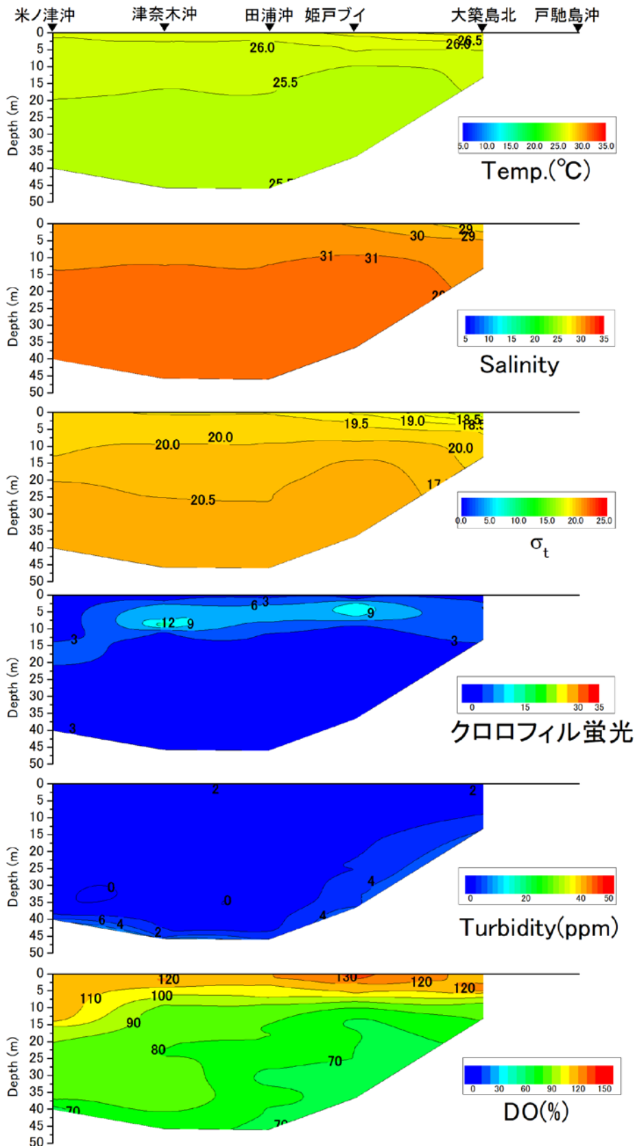
戸馳島沖から米ノ津沖の水温 (°C)、塩分、密度 ( \sigma_t )、クロロフィル蛍光強度、濁度、溶存酸素飽和度 (DO%) の鉛直面図 (熊本県水産研究センターの調査による) (2021年9月21日)
