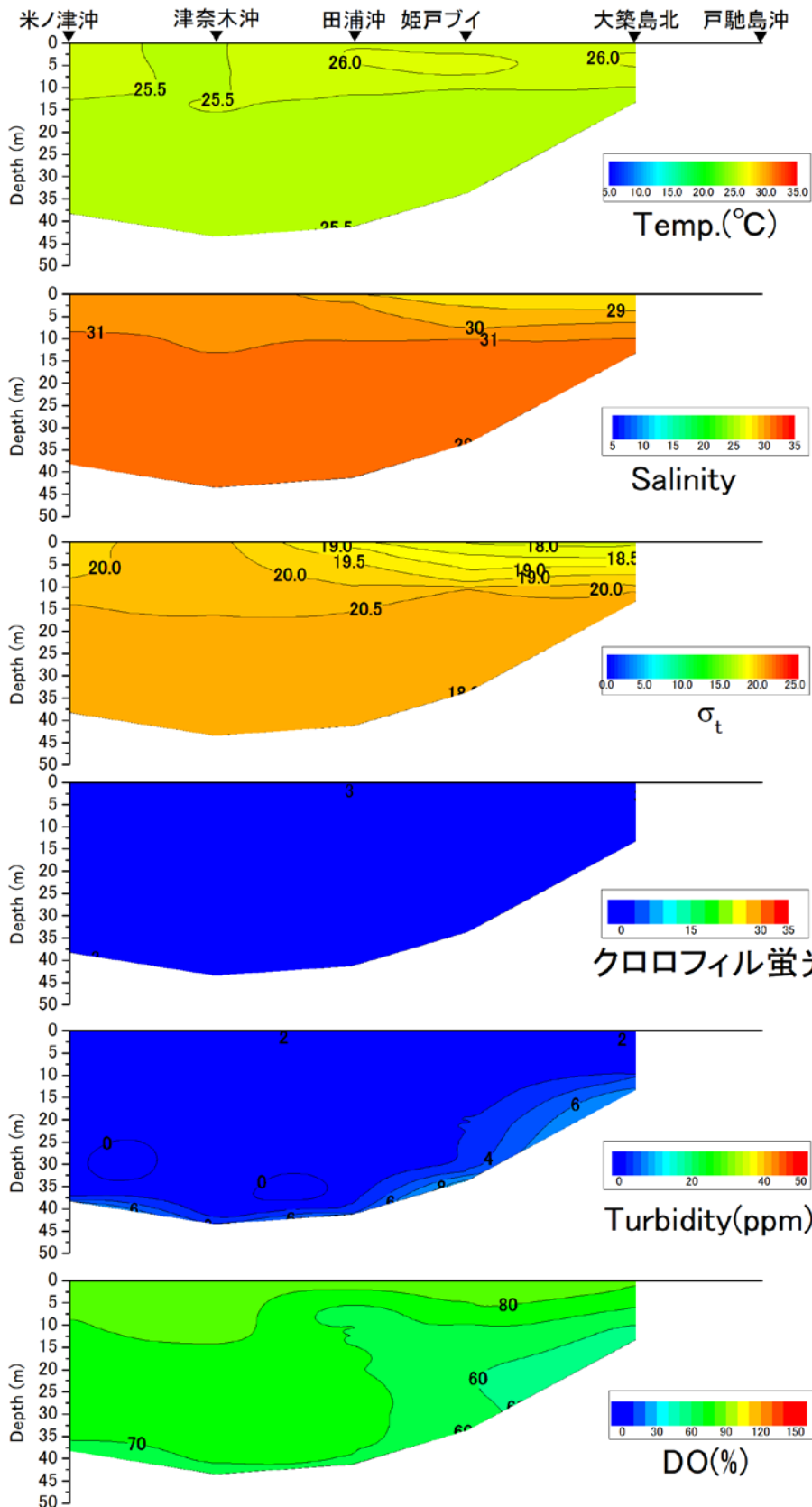
戸馳島沖から米ノ津沖の水温(°C)、塩分、密度( \sigma_t )、クロロフィル蛍光強度、濁度、溶存酸素飽和度(DO%)の鉛直面図(鹿児島県水産技術開発センターの調査による)(2021年9月14日)
