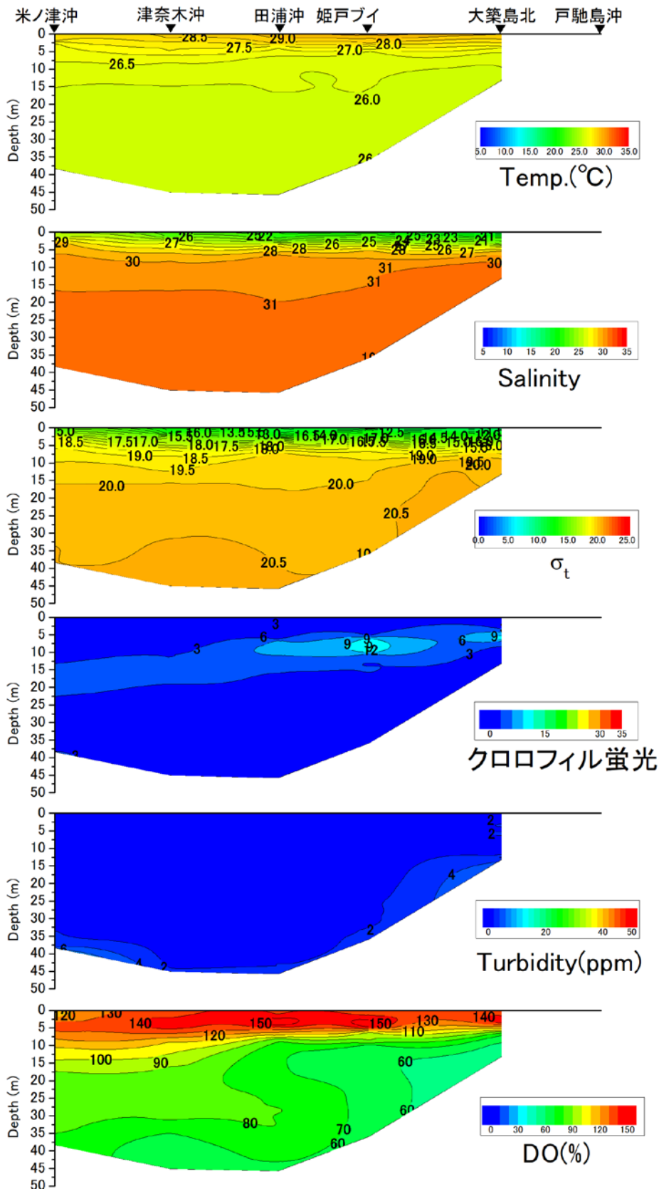
戸馳島沖から米ノ津沖の水温 (°C)、塩分、密度 ( \sigma_t )、クロロフィル蛍光強度、濁度、溶存酸素飽和度 (DO%) の鉛直面図 (熊本県水産研究センターの調査による) (2021年8月30日)
