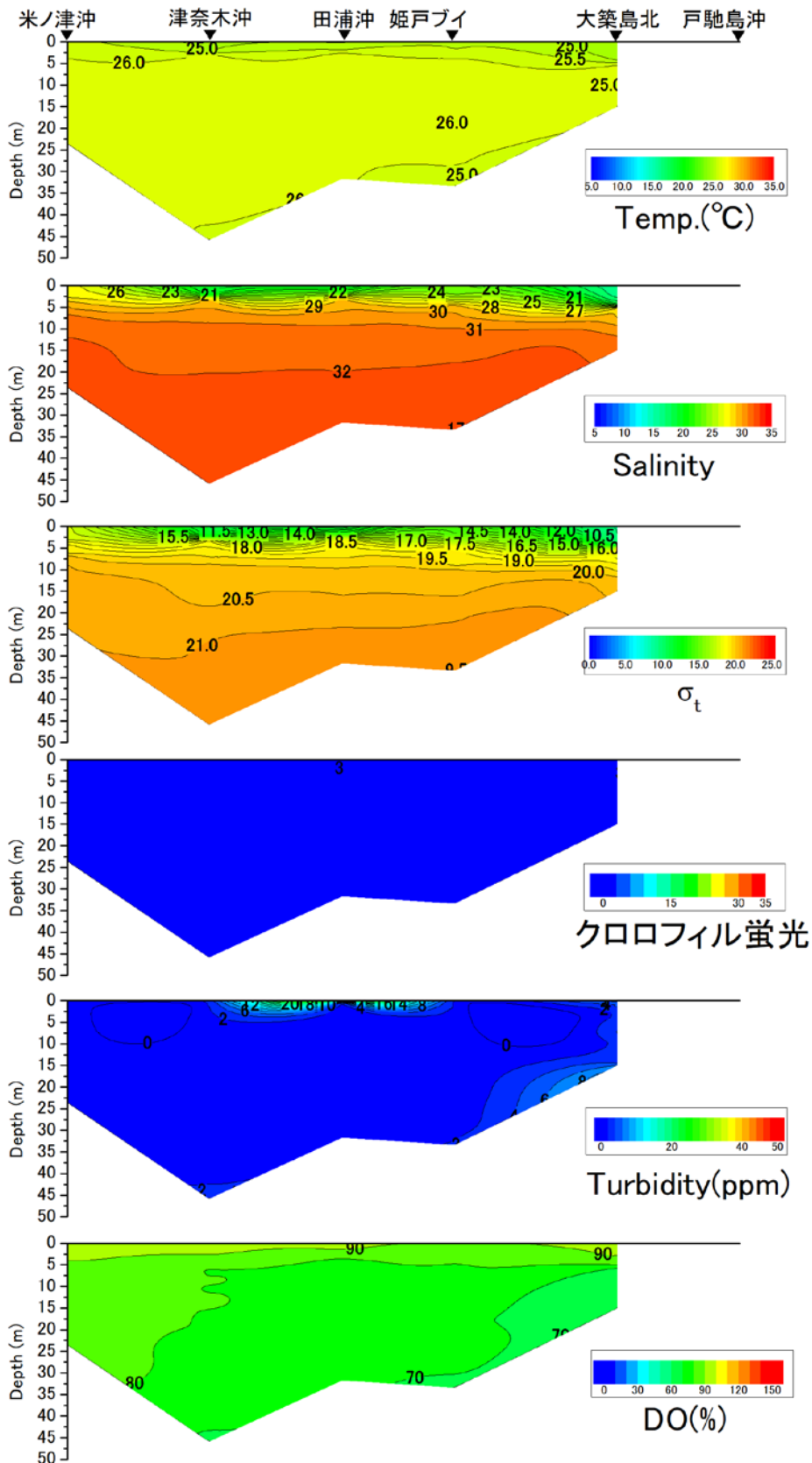
戸馳島沖から米ノ津沖の水温 (°C)、塩分、密度 ( \sigma_t )、クロロフィル蛍光強度、濁度、溶存酸素飽和度 (DO%) の鉛直面図 (東町漁業協同組合の調査による) (2021年8月17日)
