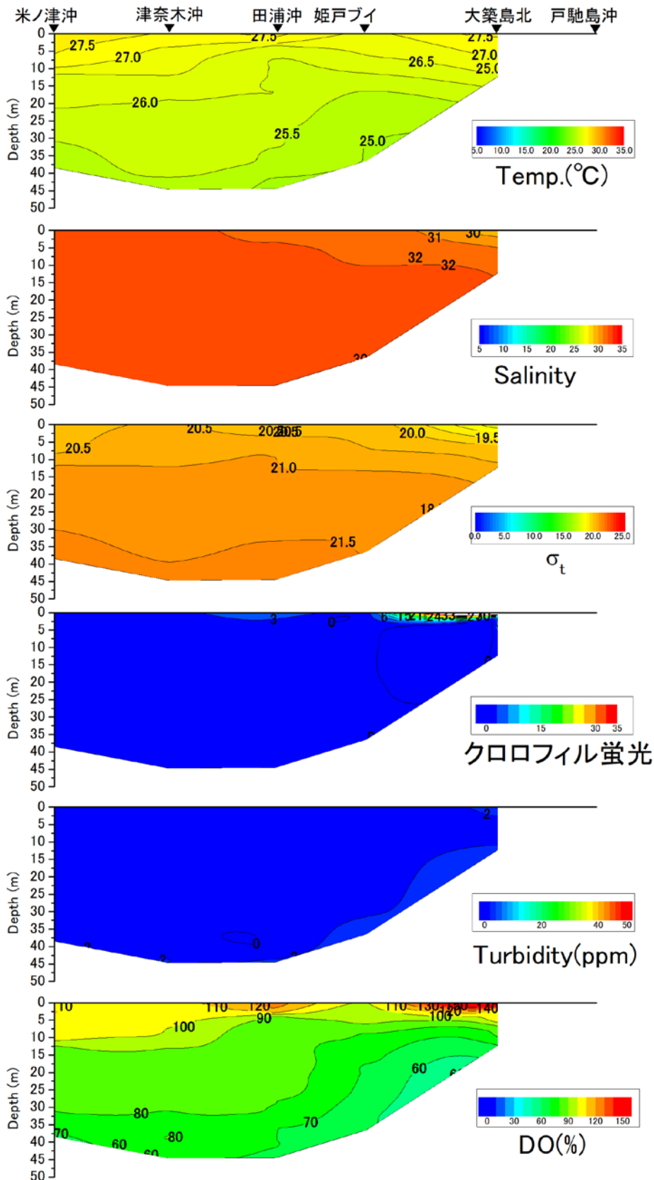
戸馳島沖から米ノ津沖の水温 (°C) 、塩分、密度 ( \sigma_t ) 、クロロフィル蛍光強度、濁度、溶存酸素飽和度 (DO%) の鉛直面図 (熊本県水産研究センターの調査による) (2021年8月10日)
