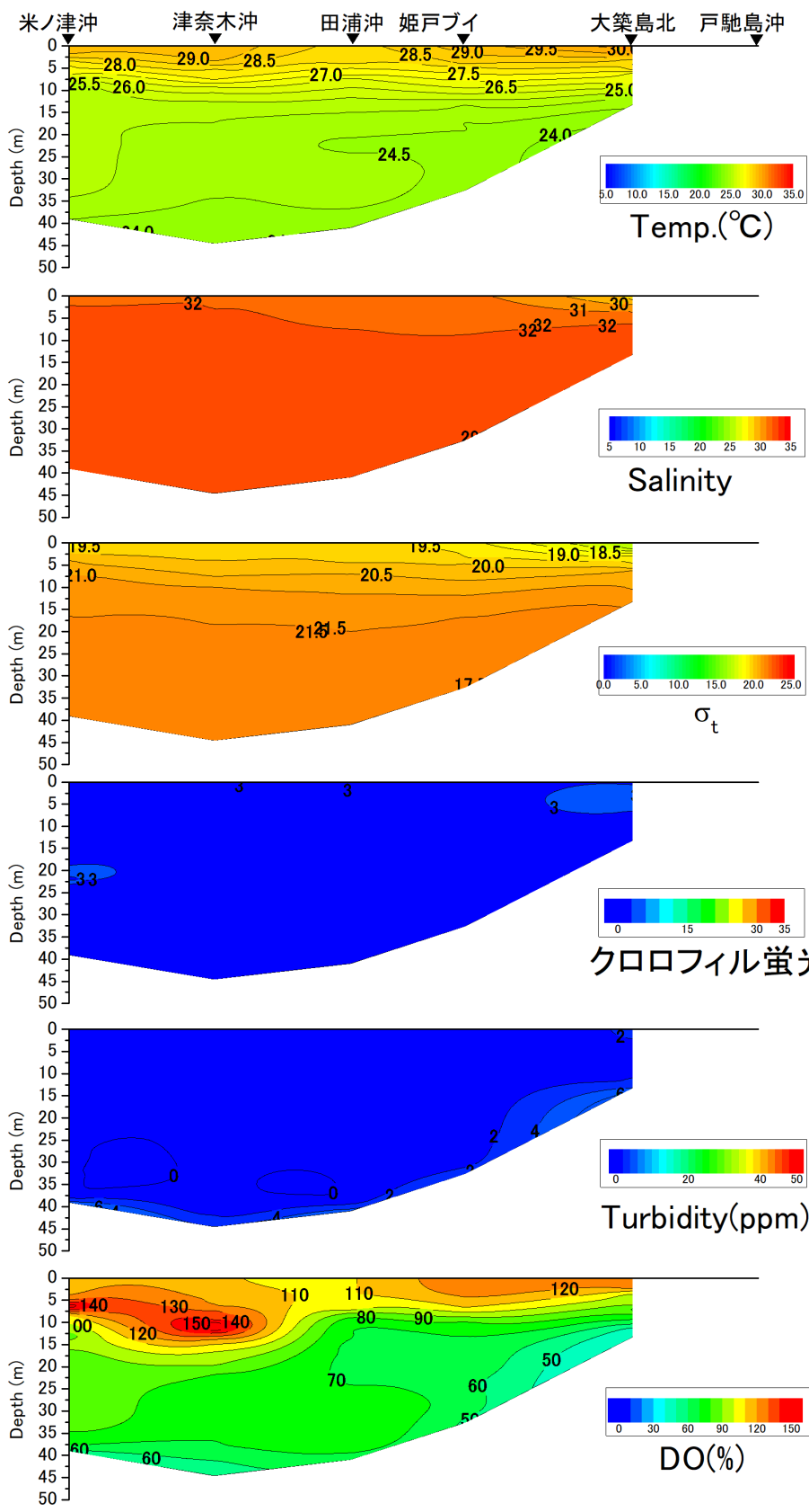
戸馳島沖から米ノ津沖の水温(°C)、塩分、密度( \sigma_t )、クロロフィル蛍光強度、濁度、溶存酸素飽和度(DO%)の鉛直面図(鹿児島県水産技術開発センターの調査による)(2021年8月3日)
