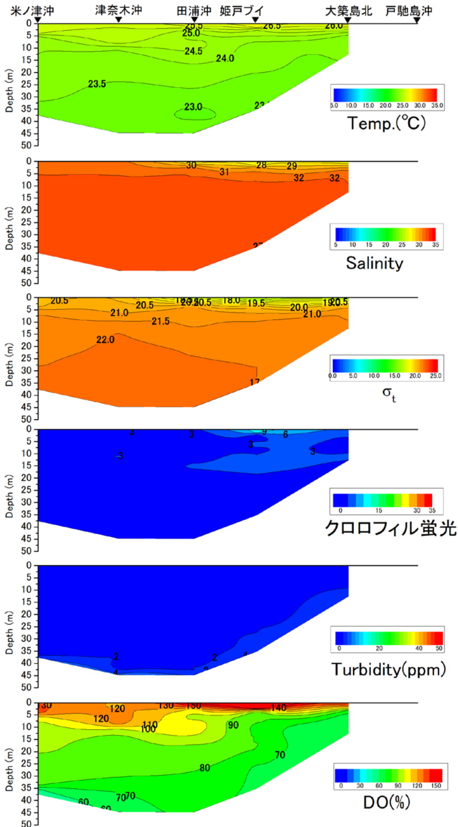
戸馳島沖から米ノ津沖の水温 (°C)、塩分、密度 ( \sigma_t )、クロロフィル蛍光強度、濁度、溶存酸素飽和度 (DO%) の鉛直面図 (熊本県水産研究センターの調査による) (2021年7月20日)
