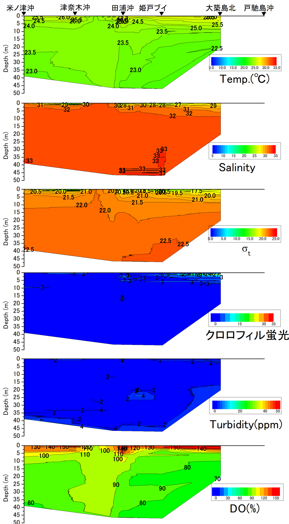
戸馳島沖から米ノ津沖の水温 (°C)、塩分、密度 ( \sigma_t )、クロロフィル蛍光強度、濁度、溶存酸素飽和度 (DO%) の鉛直面図 (東町漁業協同組合の調査による) (2021年7月13日)
