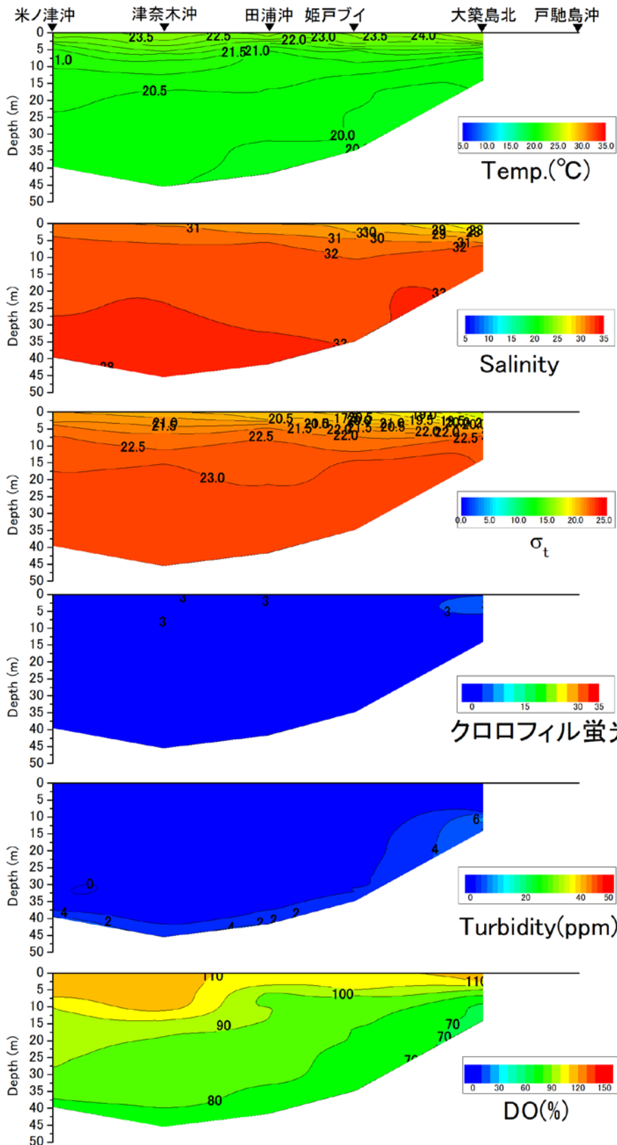
戸馳島沖から米ノ津沖の水温(°C)、塩分、密度( \sigma_t )、クロロフィル蛍光強度、濁度、溶存酸素飽和度(DO%)の鉛直面図(鹿児島県水産技術開発センターの調査による)(2021年6月15日)
