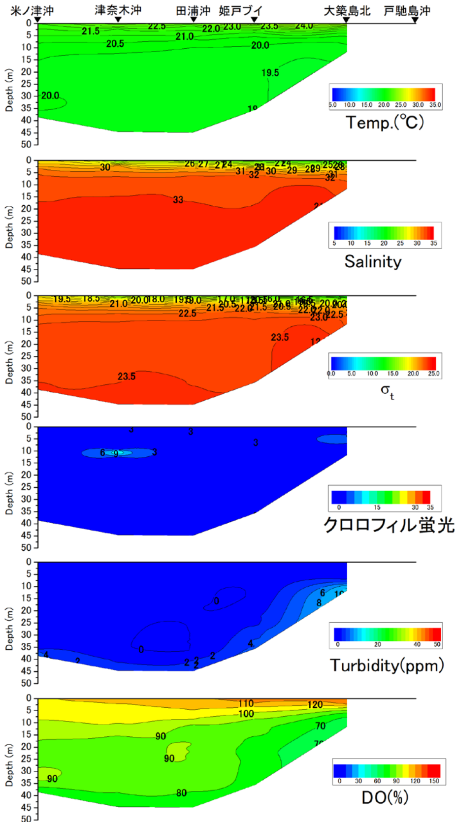
戸馳島沖から米ノ津沖の水温 (°C)、塩分、密度 ( \sigma_t )、クロロフィル蛍光強度、濁度、溶存酸素飽和度 (DO%) の鉛直面図 (熊本県水産研究センターの調査による) (2021年6月8日)
