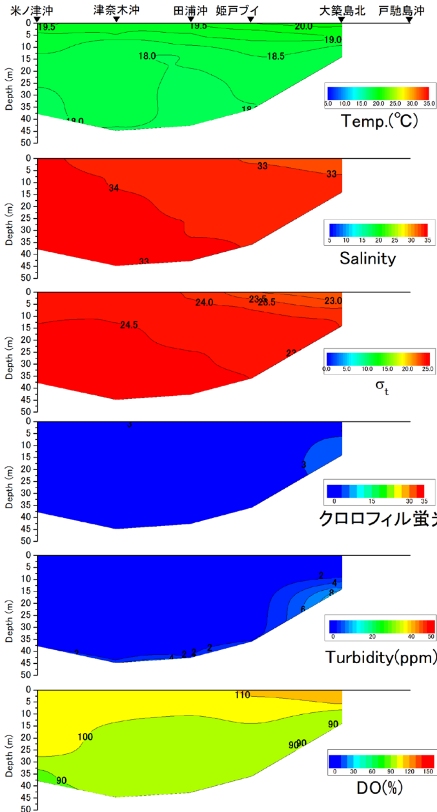
戸馳島沖から米ノ津沖の水温(°C)、塩分、密度( \sigma_t )、クロロフィル蛍光強度、濁度、溶存酸素飽和度(DO%)の鉛直面図(鹿児島県水産技術開発センターの調査による)(2021年5月11日)
