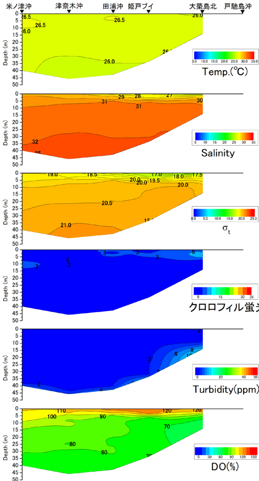
戸馳島沖から米ノ津沖の水温(°C)、塩分、密度( \sigma_t )、クロロフィル蛍光強度、濁度、溶存酸素飽和度(DO%)の鉛直面図(鹿児島県水産技術開発センターの調査による)(2020年9月15日)
