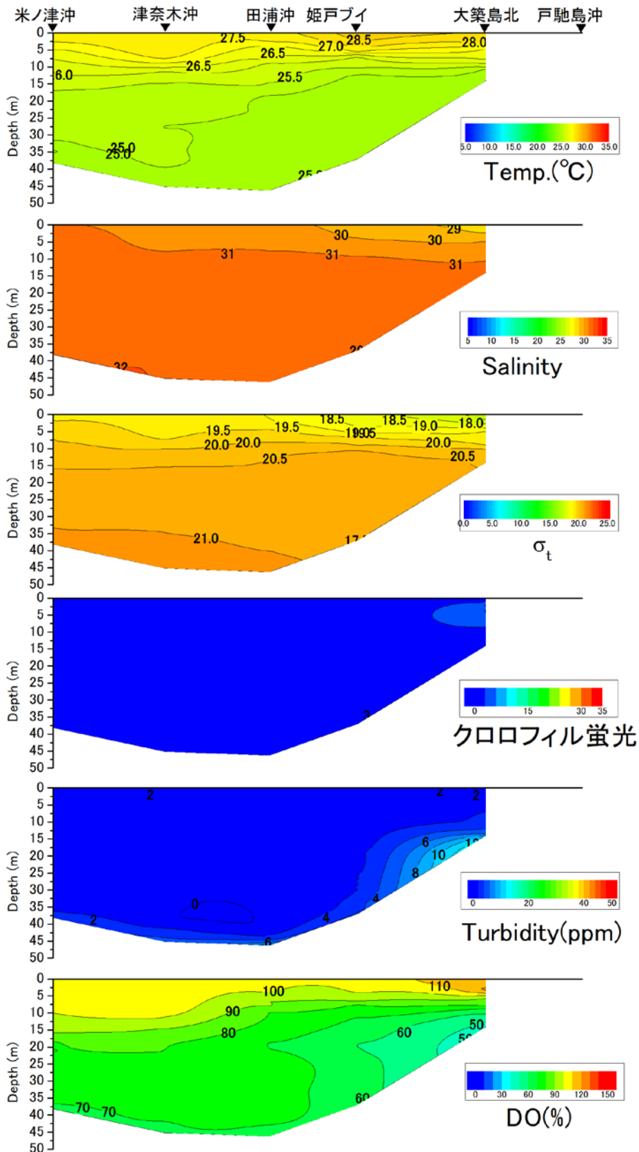
戸馳島沖から米ノ津沖の水温 (°C)、塩分、密度 ( \sigma_t )、クロロフィル蛍光強度、濁度、溶存酸素飽和度 (DO%) の鉛直面図 (熊本県水産研究センターの調査による) (2020年8月31日)
