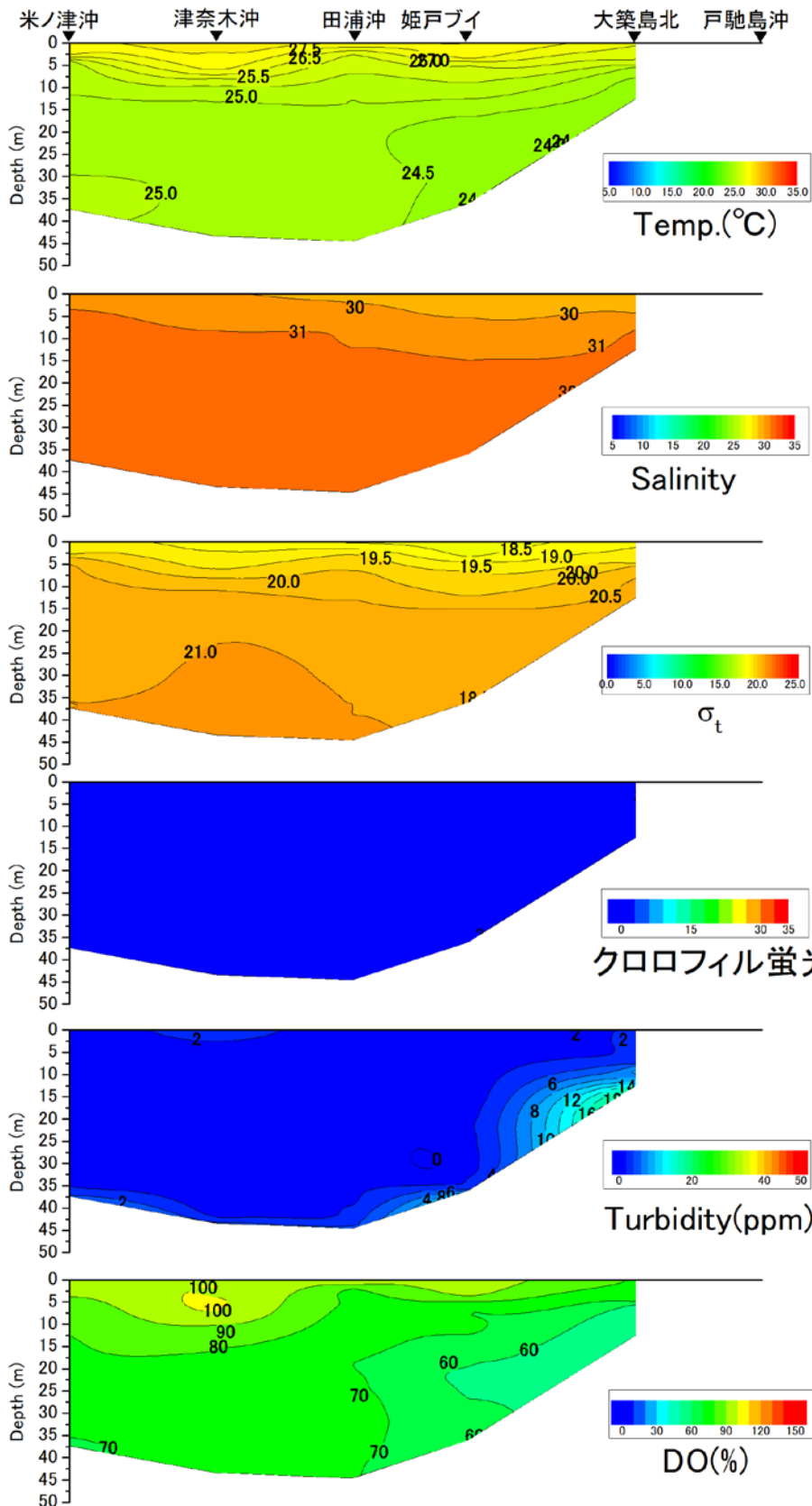
戸馳島沖から米ノ津沖の水温(°C)、塩分、密度( \sigma_t )、クロロフィル蛍光強度、濁度、溶存酸素飽和度(DO%)の鉛直面図(鹿児島県水産技術開発センターの調査による)(2020年8月25日)
