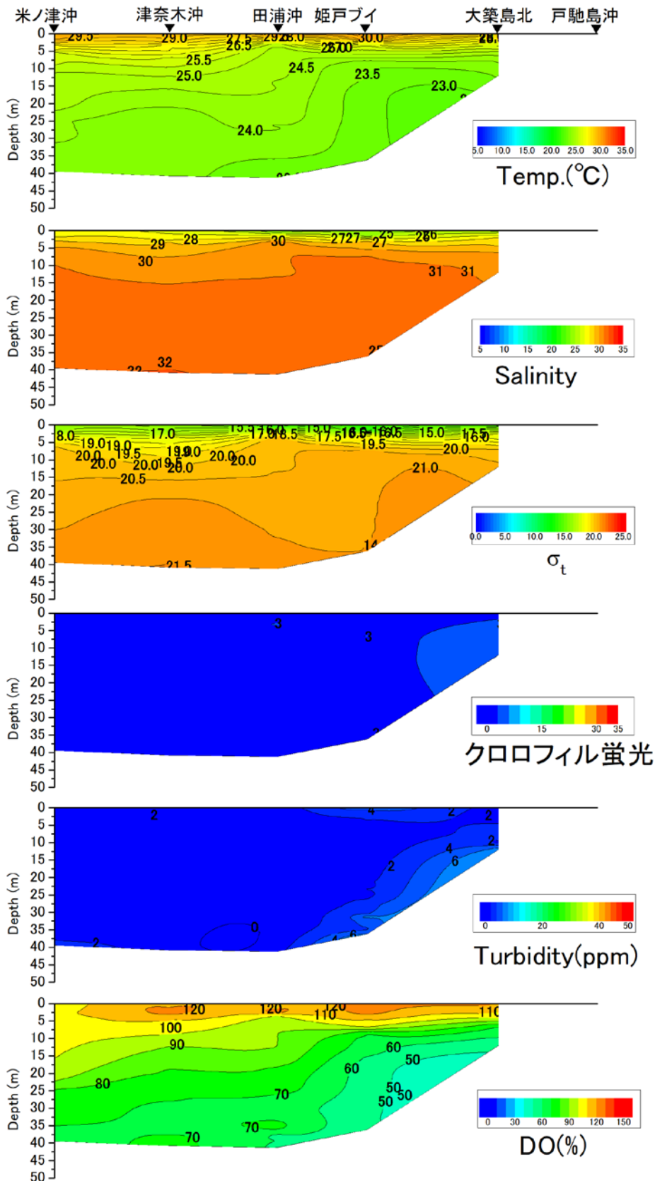
戸馳島沖から米ノ津沖の水温 (°C)、塩分、密度 ( \sigma_t )、クロロフィル蛍光強度、濁度、溶存酸素飽和度 (DO%) の鉛直面図 (東町漁業協同組合の調査による) (2020年8月18日)
